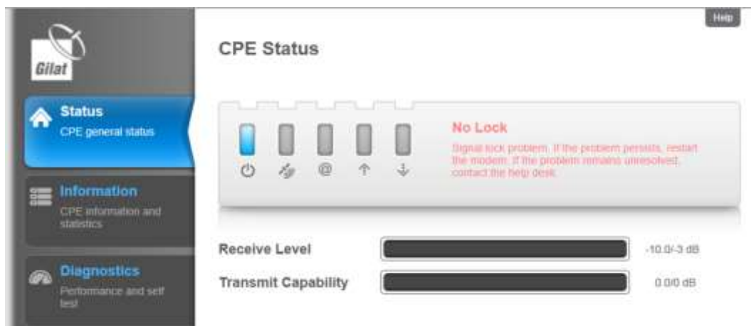
Fig 21 CPE Status Antena Desapuntada.
