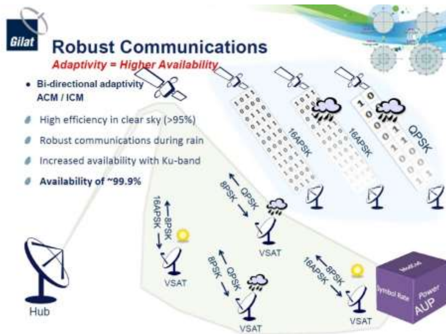
Fig 15 Codificación y Modulación Adaptativa (ACM).
