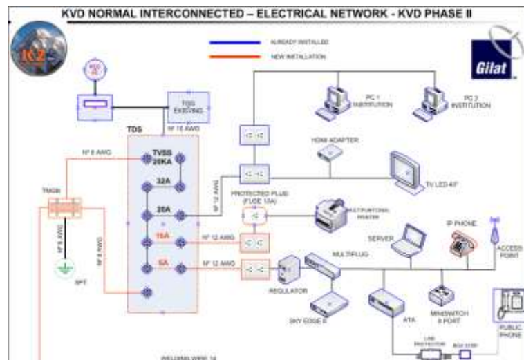
Fig 25 KVD Interconectado
