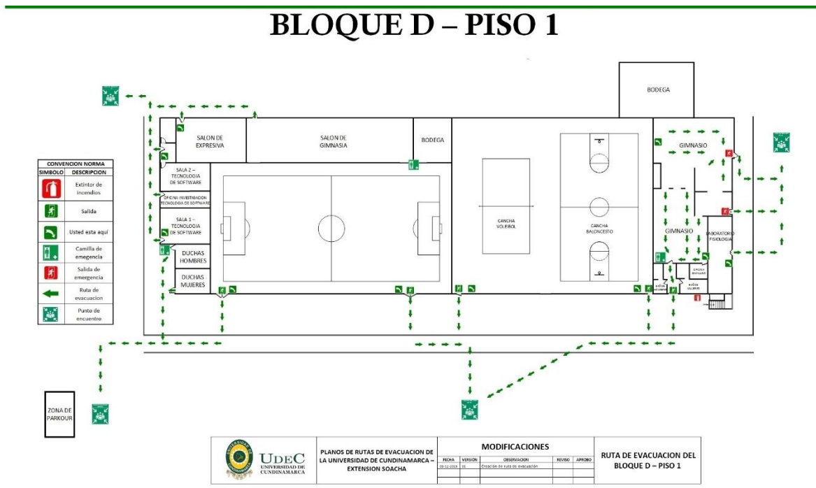
Figura 4 Plano Bloque de piso 1
