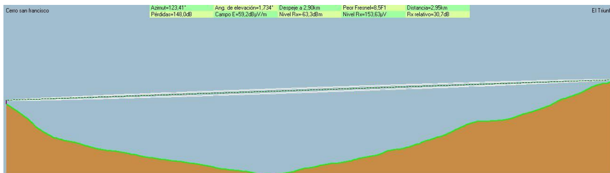
Figura 36. Enlace Cerro San Francisco – El Triunfo
