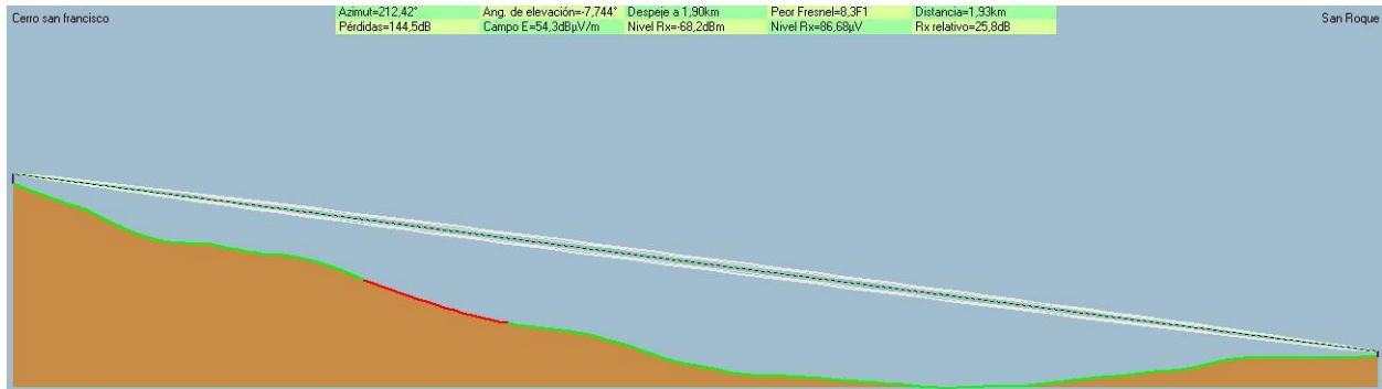
Figura 30. Enlace Cerro San Francisco – San Roque
