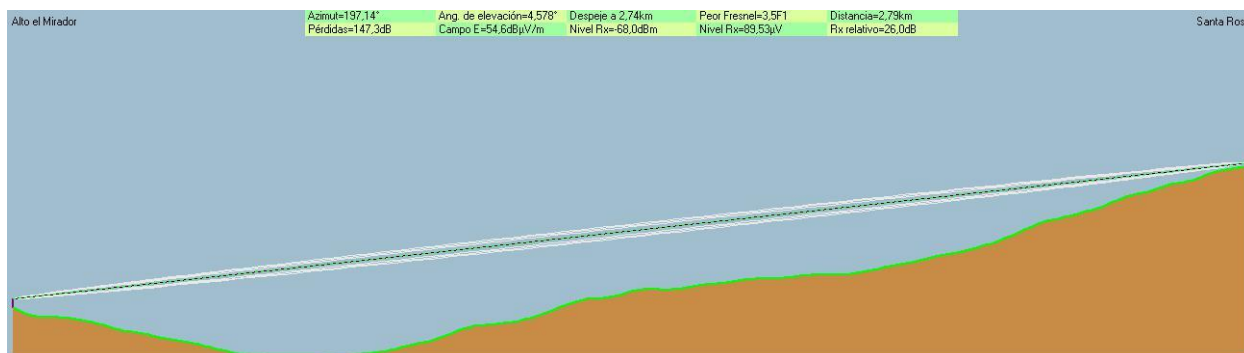
Figura 55. Enlace Alto el Mirador – Santa Rosa
