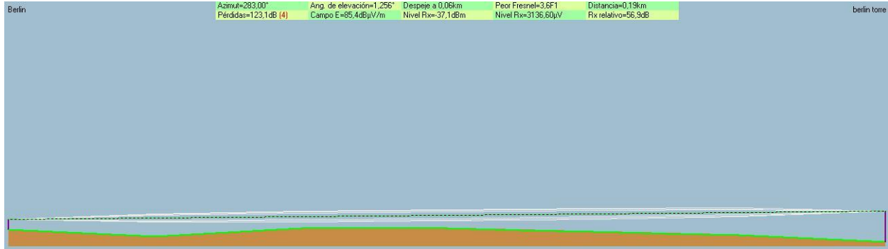
Figura 22. Enlace Torre Berlín- Berlín
