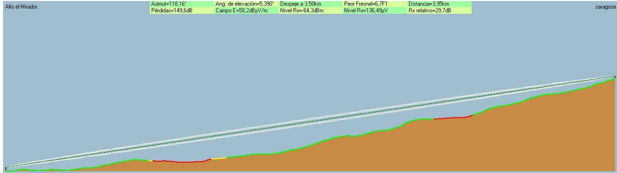
Figura 44. Enlace Alto el Mirador – Zaragoza
