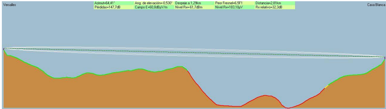
Figura 57. Enlace Versalles – Casa Blanca
