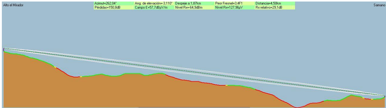
Figura 42. Enlace Alto el Mirador – EL Sámano
