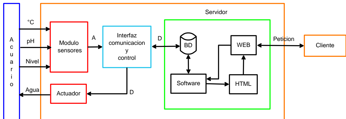
Figura 2 Diagrama en Bloques del sistema
