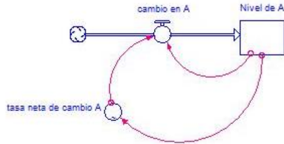
Ilustración 138 Diagrama Forrester. Modelo de Autoreferencia Fuente: Elaboración propia, Screenshot of software Stella
