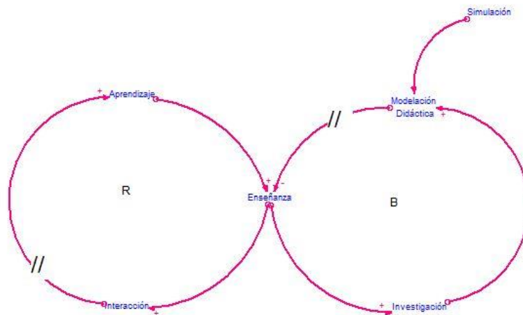
Ilustración 113 Arquetipo – Límite del crecimiento Fuente: Elaboración Propia, Screenshot of software Stella
