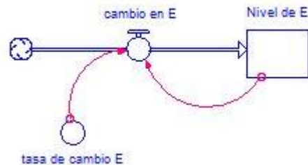
Ilustración 130 Diagrama Forrester. Modelo Exponencial Fuente: Elaboración propia, Screenshot of software Stella
