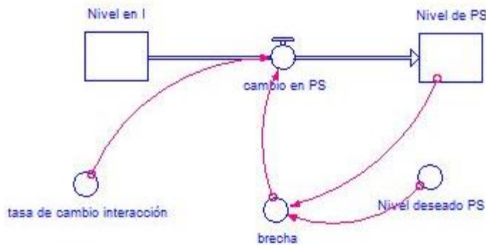
Ilustración 105 Diagrama de Forrester. Subsistema INVESTIGACIÓN – PROYECCIÓN SOCIAL Fuente: Elaboración Propia, Screenshot of software Stella
