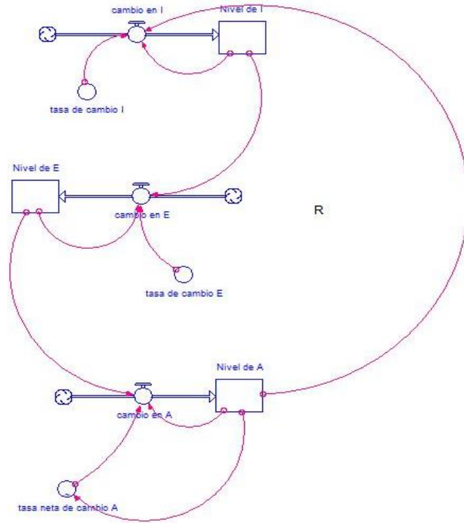
Ilustración 80 Diagrama de Forrester. Subsistema ENSEÑANZA-APRENDIZAJE- INVESTIGACIÓN Fuente: Elaboración propia, Screenshot of software Stella
