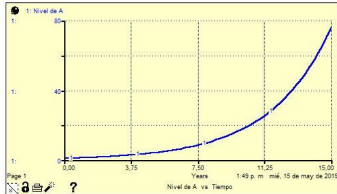
Ilustración 135 Patrón de comportamiento en el tiempo. Curva de crecimiento exponencial Fuente: Elaboración propia, Screenshot of software Stella
