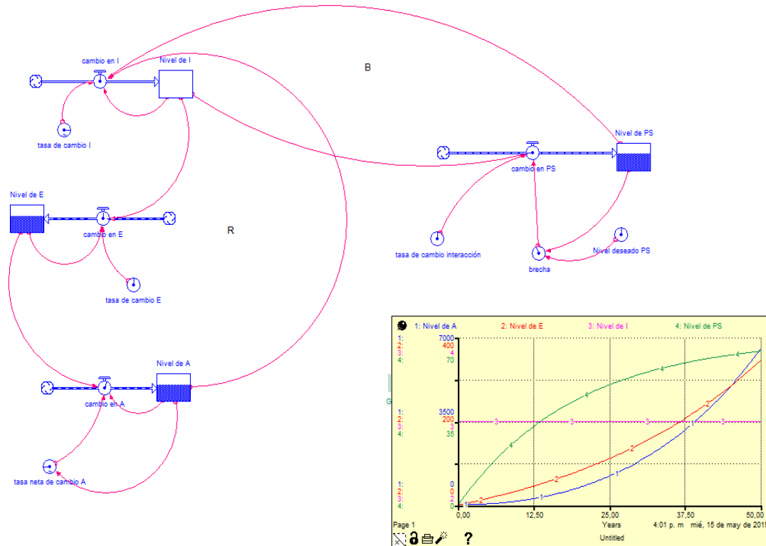
Ilustración 148 Diagrama Forrester y Patrones de Comportamiento del Sistema EAIPS
