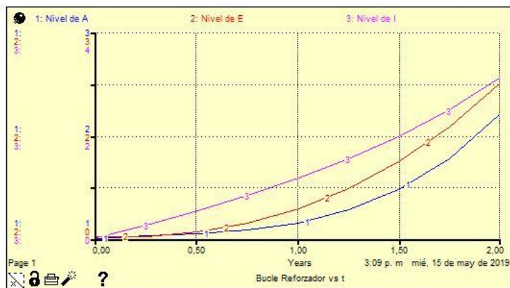
Ilustración 81 Patrón de Conducta en el tiempo – Subsistema ENSEÑANZA-APRENDIZAJE- INVESTIGACIÓN Fuente: Elaboración propia, Screenshot of software Stella
