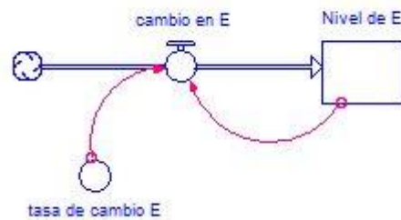
Ilustración 71 Diagrama de Forrester- Categoría ENSEÑANZA. Modelo exponencial Fuente: Elaboración propia, Screenshot of software Stella
