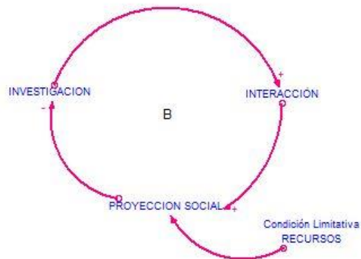
Ilustración 124 Diagrama Causal. Bucle Compensador Fuente: Elaboración propia, Screenshot of software Stella
