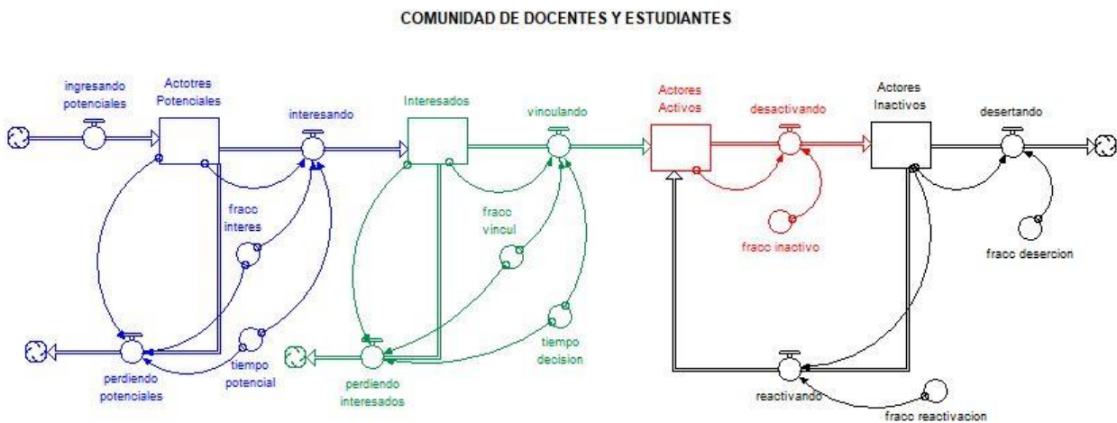
Ilustración 116 Diagrama de Stock y Flujo – Proceso de Interacción Fuente: Elaboración Propia, Screenshot of software Stella
