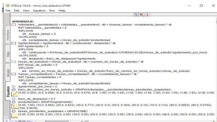
Ilustración 122 Ecuaciones en Código STELLA Fuente: Screenshot of software Stella
