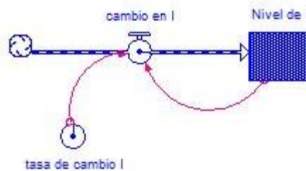
Ilustración 77 Diagrama de Forrester – Categoría INVESTIGACIÓN. Modelo Exponencial Fuente: Elaboración propia, Screenshot of software Stella
