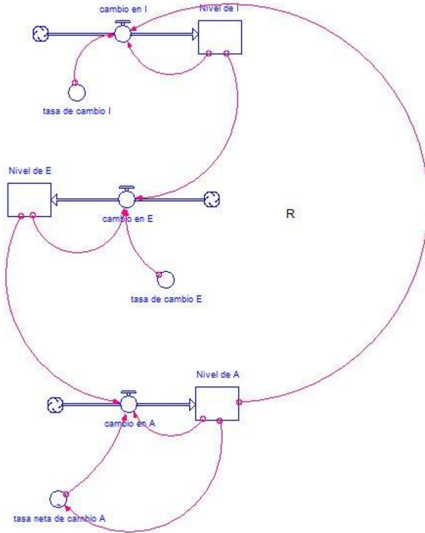
Ilustración 141 Diagrama Forrester. Subsistema EAI Fuente: Elaboración propia, Screenshot of software Stella
