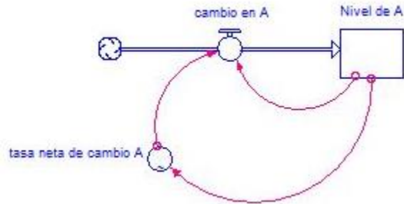
Ilustración 75 Diagrama de Forrester – Categoría APRENDIZAJE. Modelo Autoreferencia Fuente: Elaboración propia, Screenshot of software Stella
