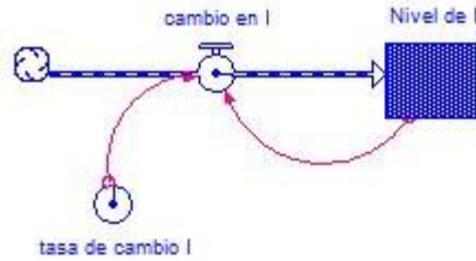
Ilustración 100 Diagrama de Forrester – Categoría INVESTIGACIÓN. Modelo Exponencial Fuente: Elaboración Propia, Screenshot of software Stella
