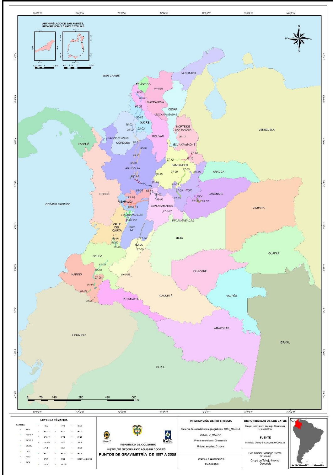
Figura 7.3. Mapa General de puntos de gravimetría. Elaboración propia.
