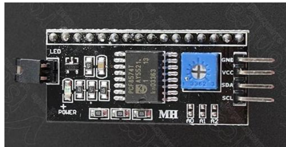
Figura 32 Placa I2C adaptadora LCD1602 Fuente: Vistronica
