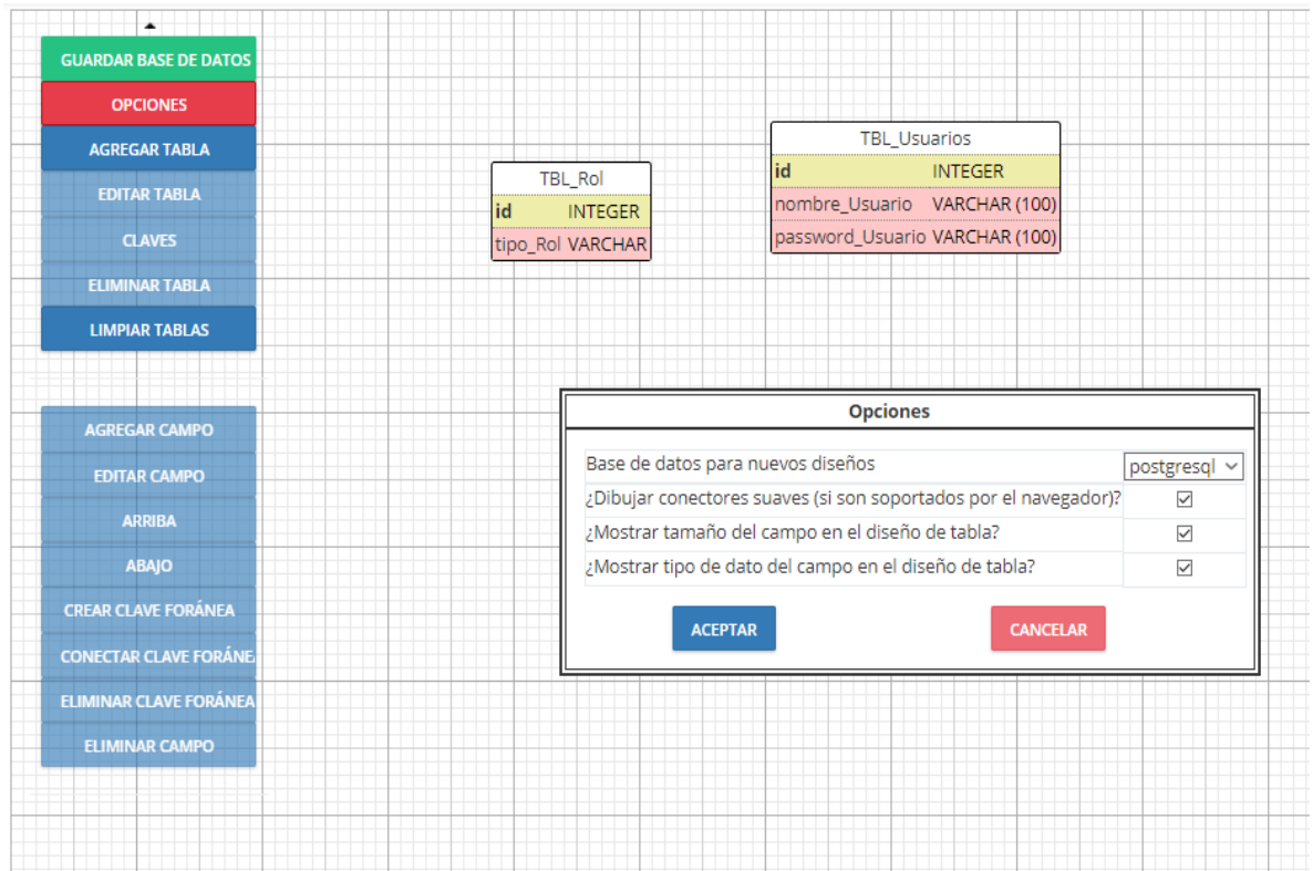
Imagen 46 Opciones del Modelo Grafico.
