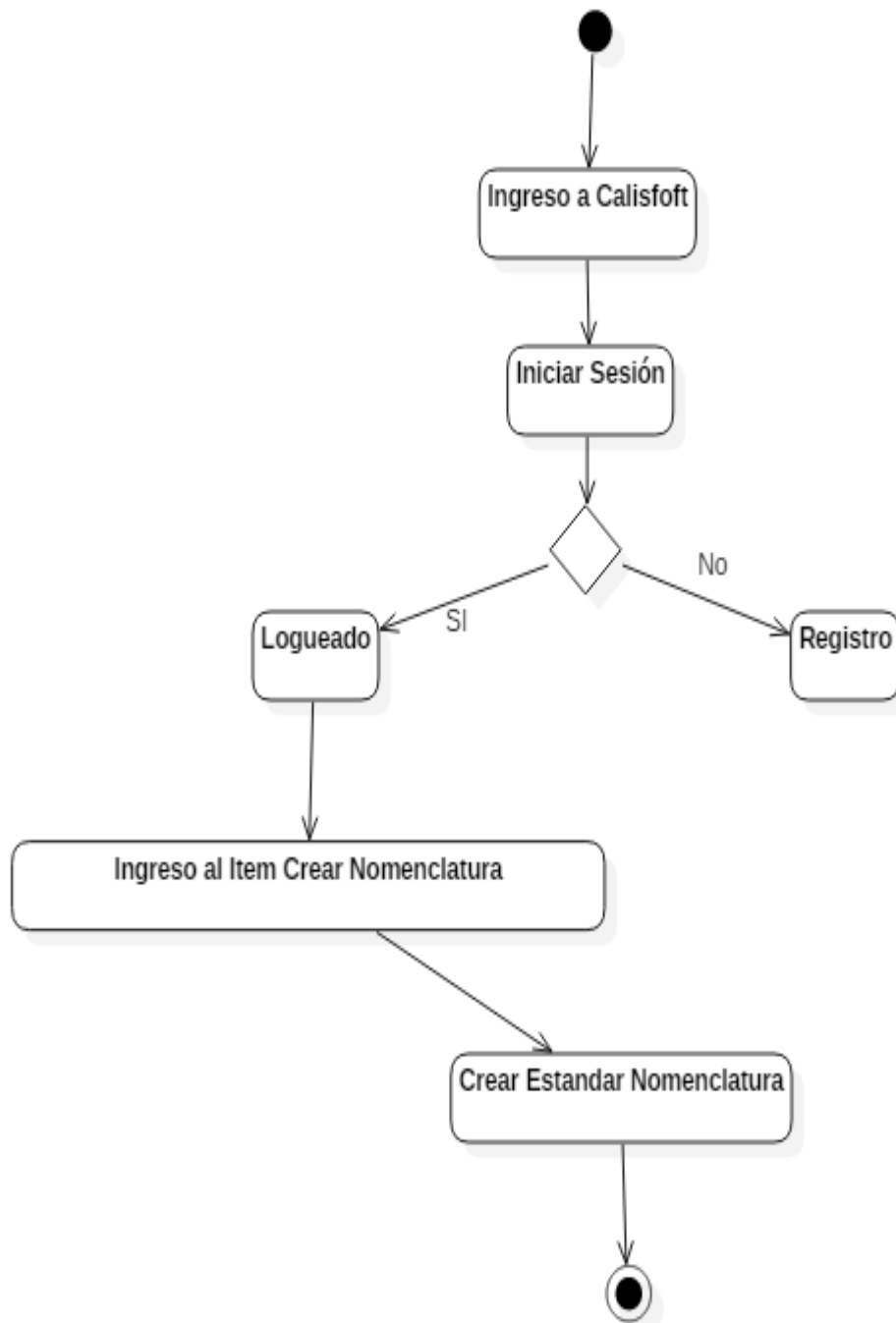
Imagen 22 Diagrama de Actividad Crear Estándares.
