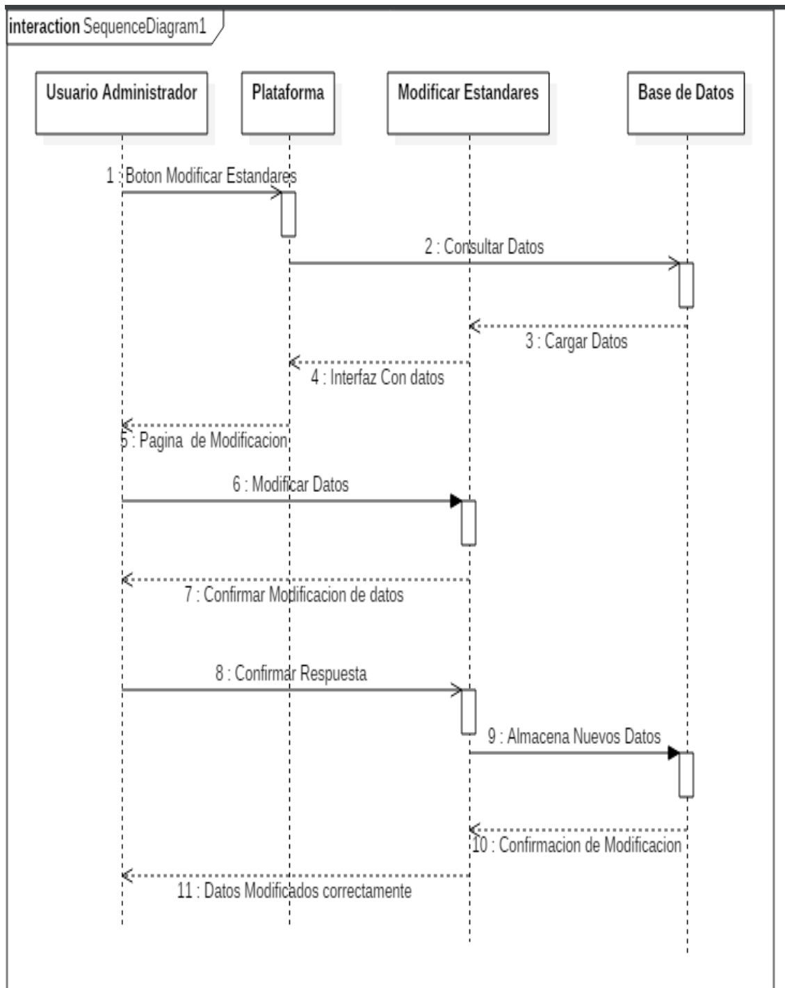
Imagen 16 Diagrama de Secuencia Modificar Estándares.
