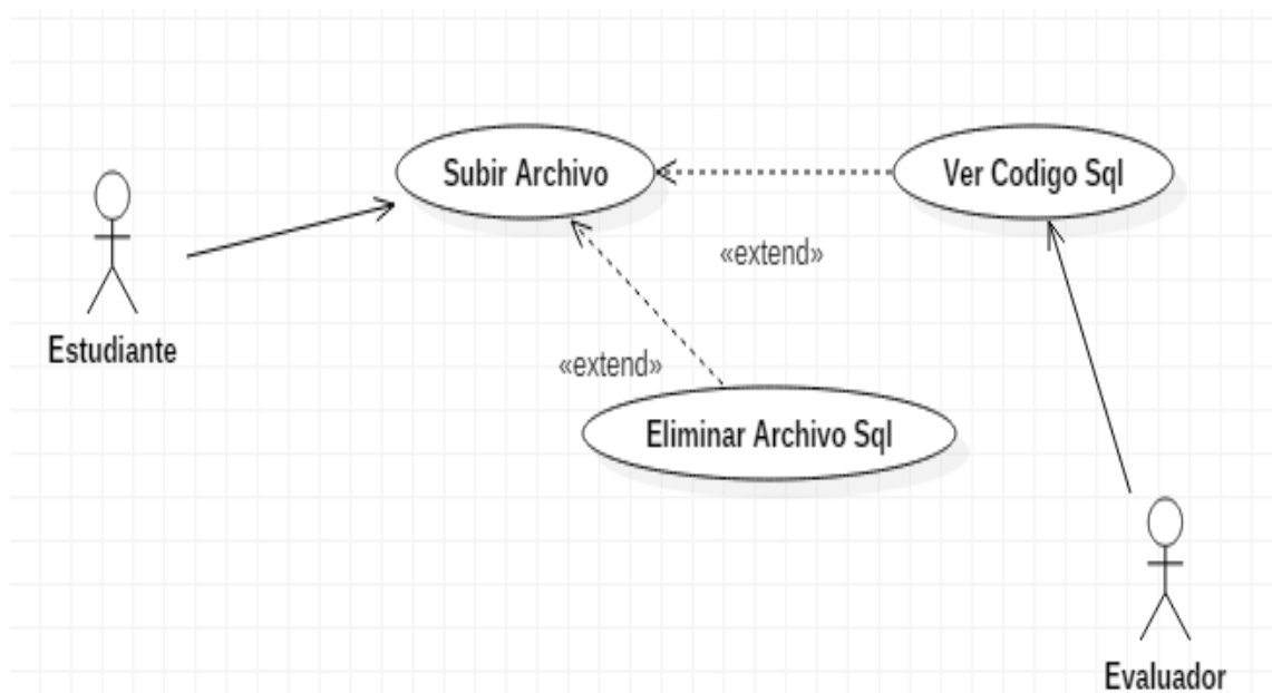
Imagen 4 Caso de Uso Subir Archivo.
