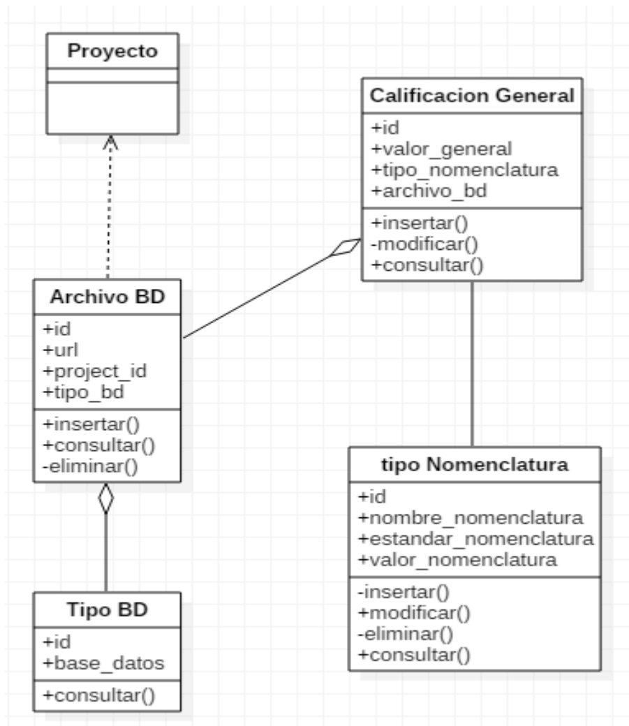
Imagen 25 Diagrama de Clases
