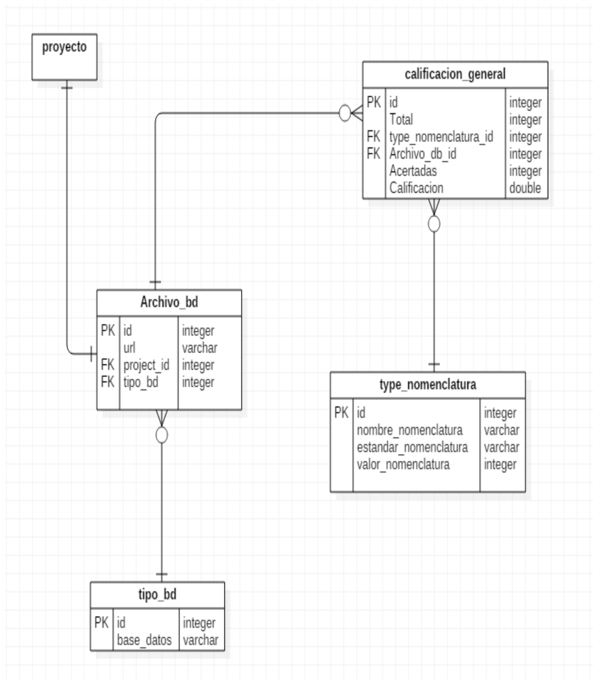
Imagen 2 Diagrama Modelo Entidad – Relación .
