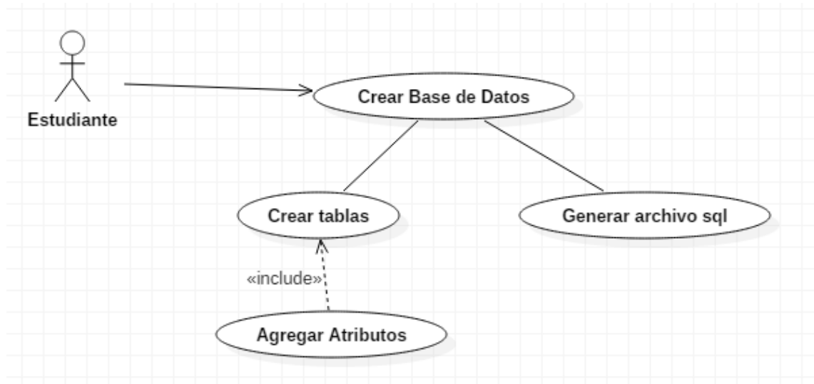
Imagen 5 Caso de Uso Crear Base de Datos.
