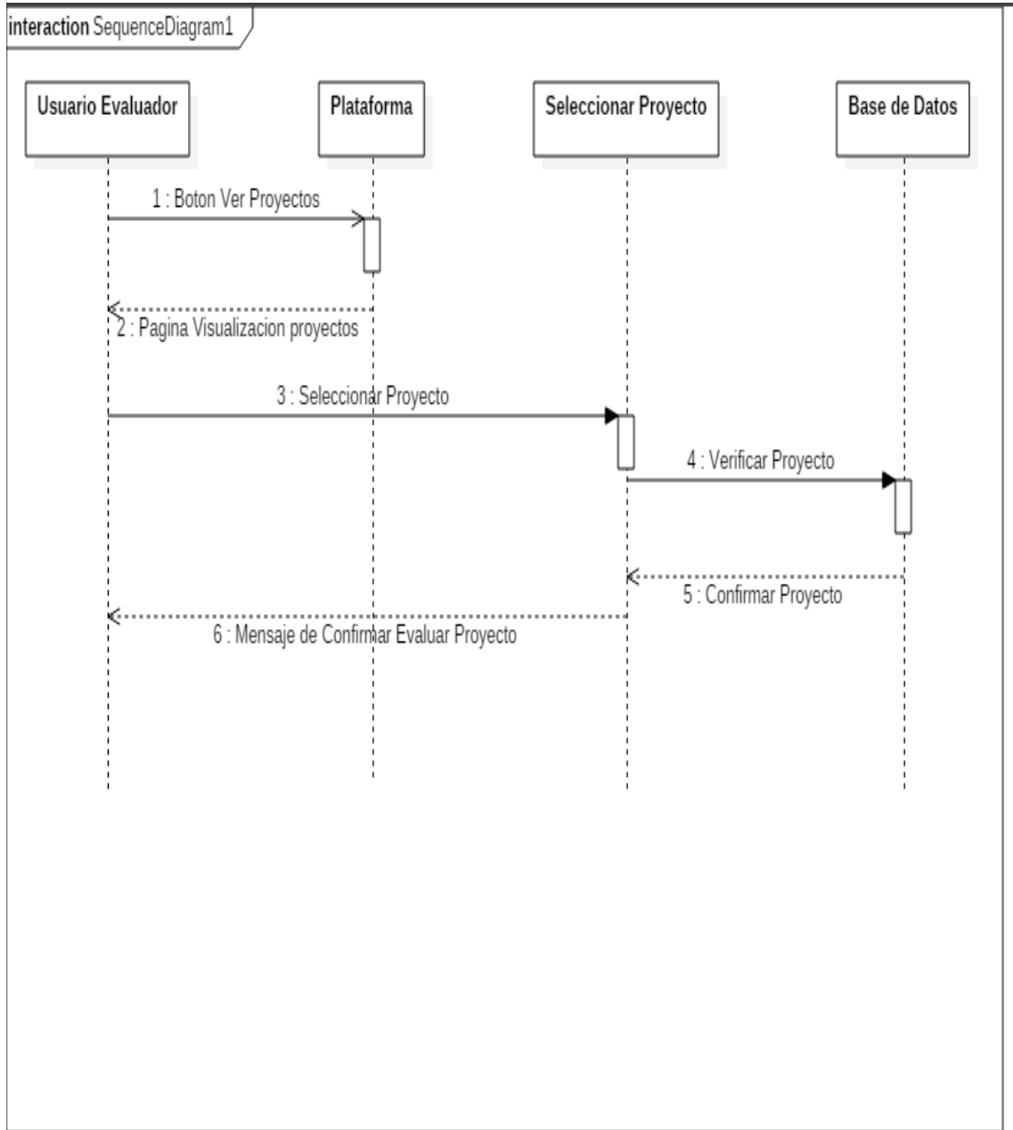
Imagen 13 Diagrama de Secuencia Seleccionar Proyecto a Evaluar.
