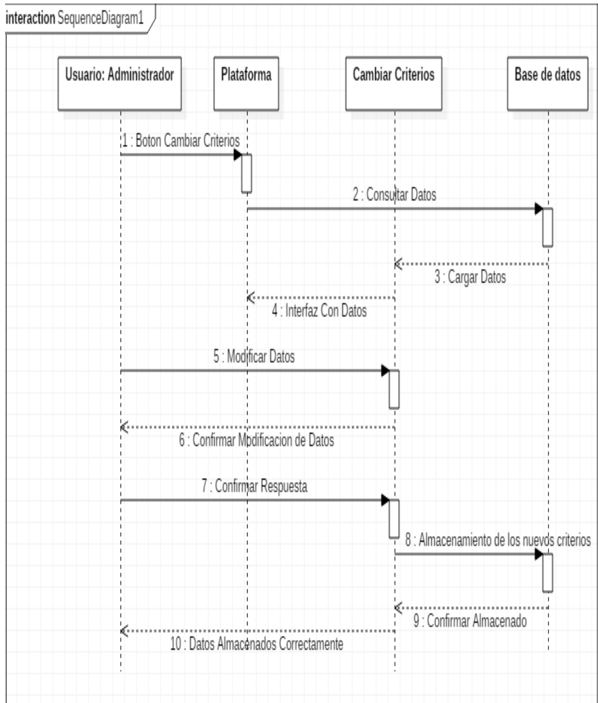
Imagen 17 Diagrama de Secuencia Cambiar Criterios de Evaluación.
