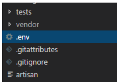
Ilustración 42 Archivo. env
