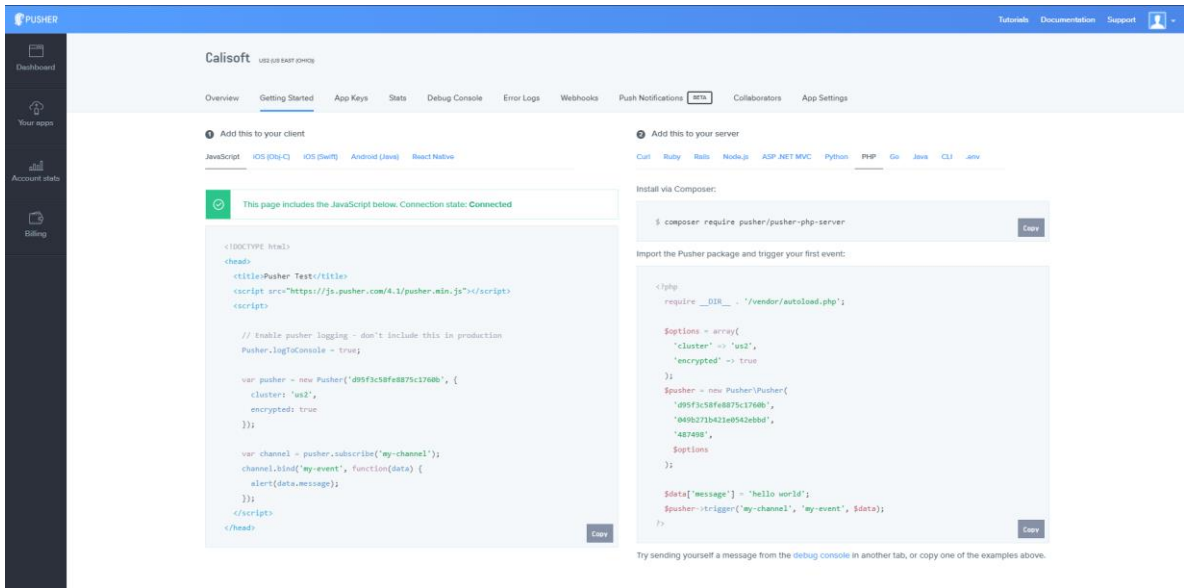
Ilustración 37 Backend Pusher
