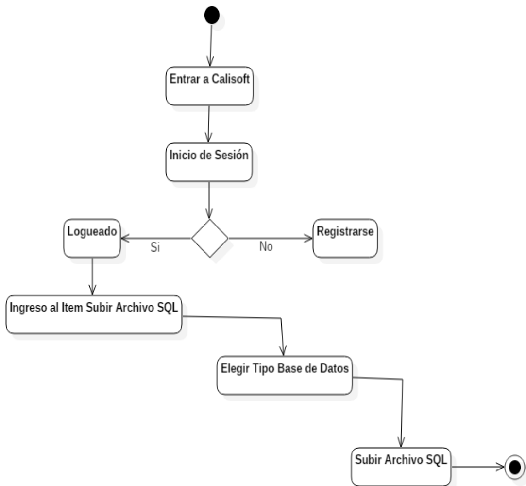
Imagen 18 Diagrama de Actividad Subir Archivo.
