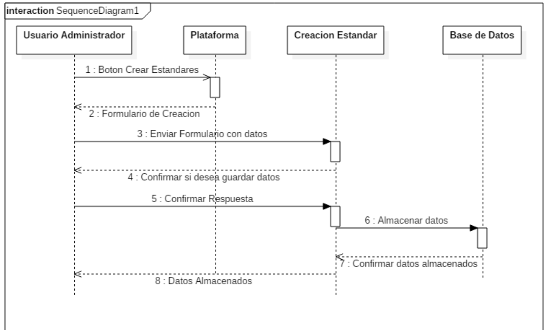
Imagen 15 Diagrama de Secuencia Crear Estándares
