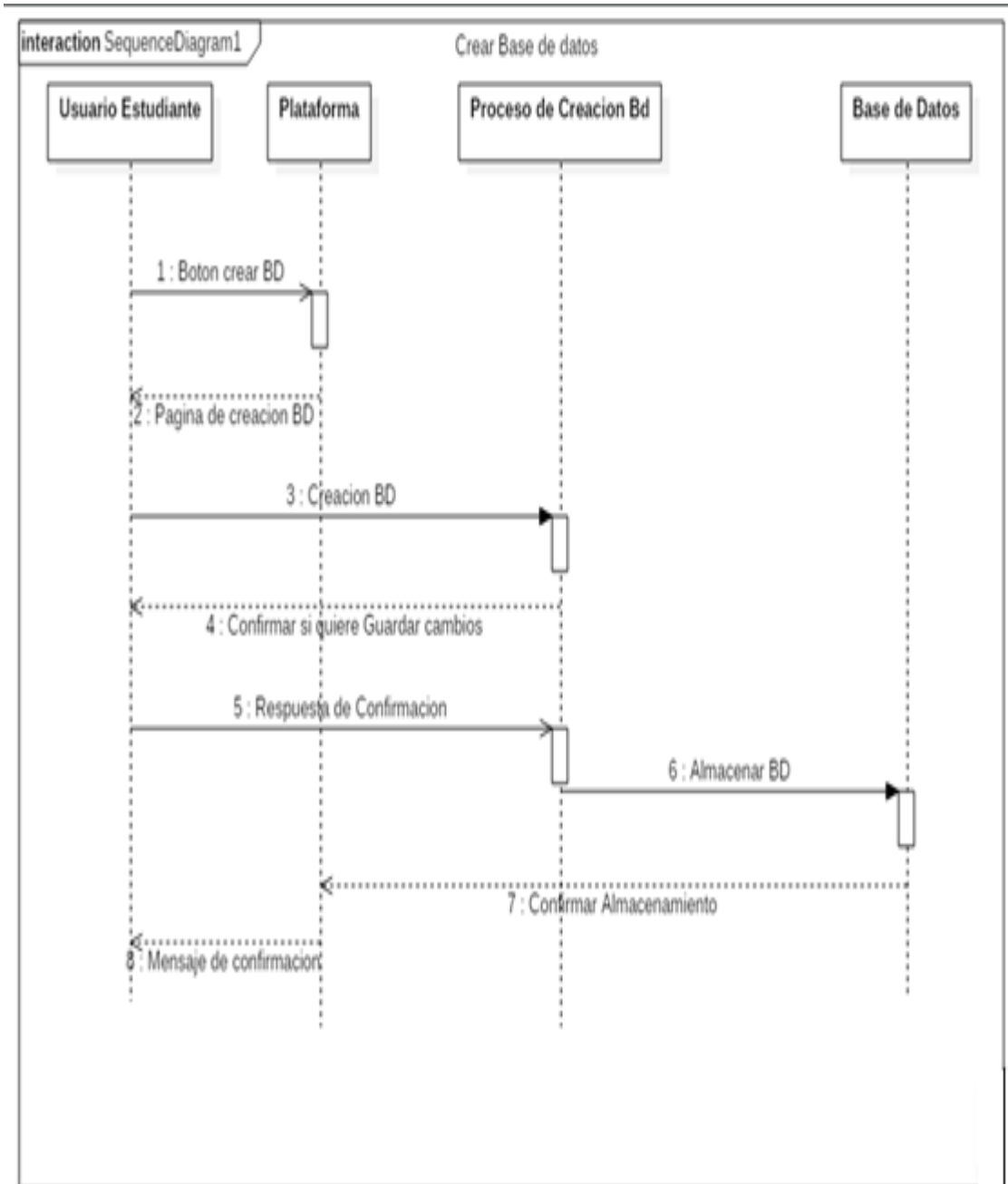
Imagen 12 Diagrama de Secuencia Crear Base de Datos.
