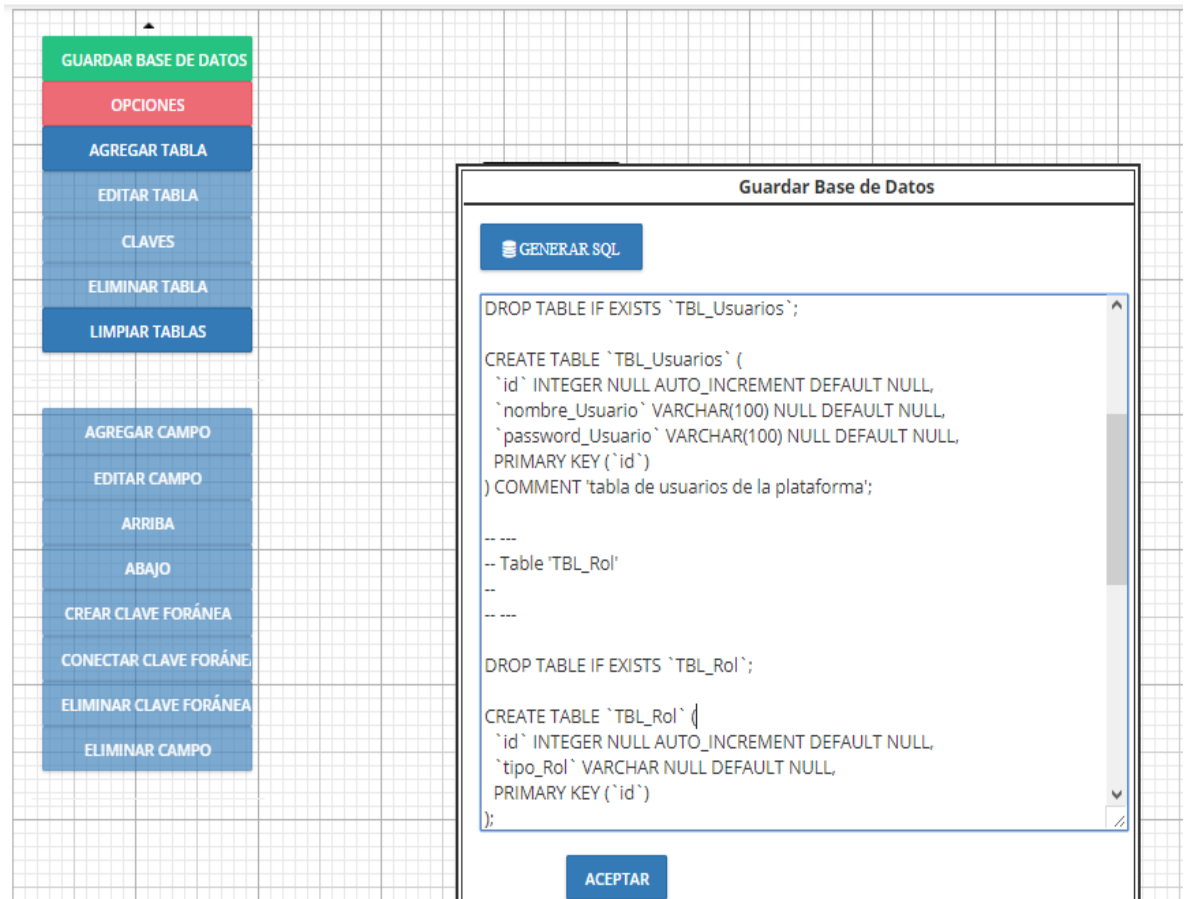
Imagen 45 Exportar Base de datos.
