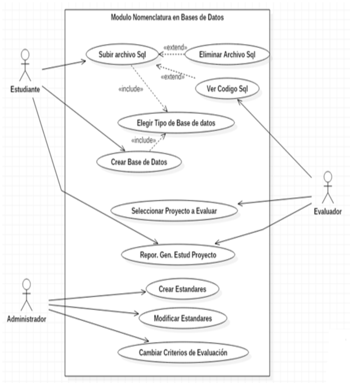
Imagen 3 Diagrama de Casos de Uso Principal.
