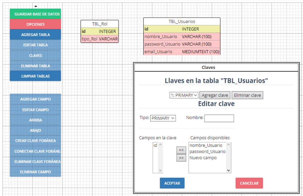
Imagen 49 Manejo de Relaciones.
