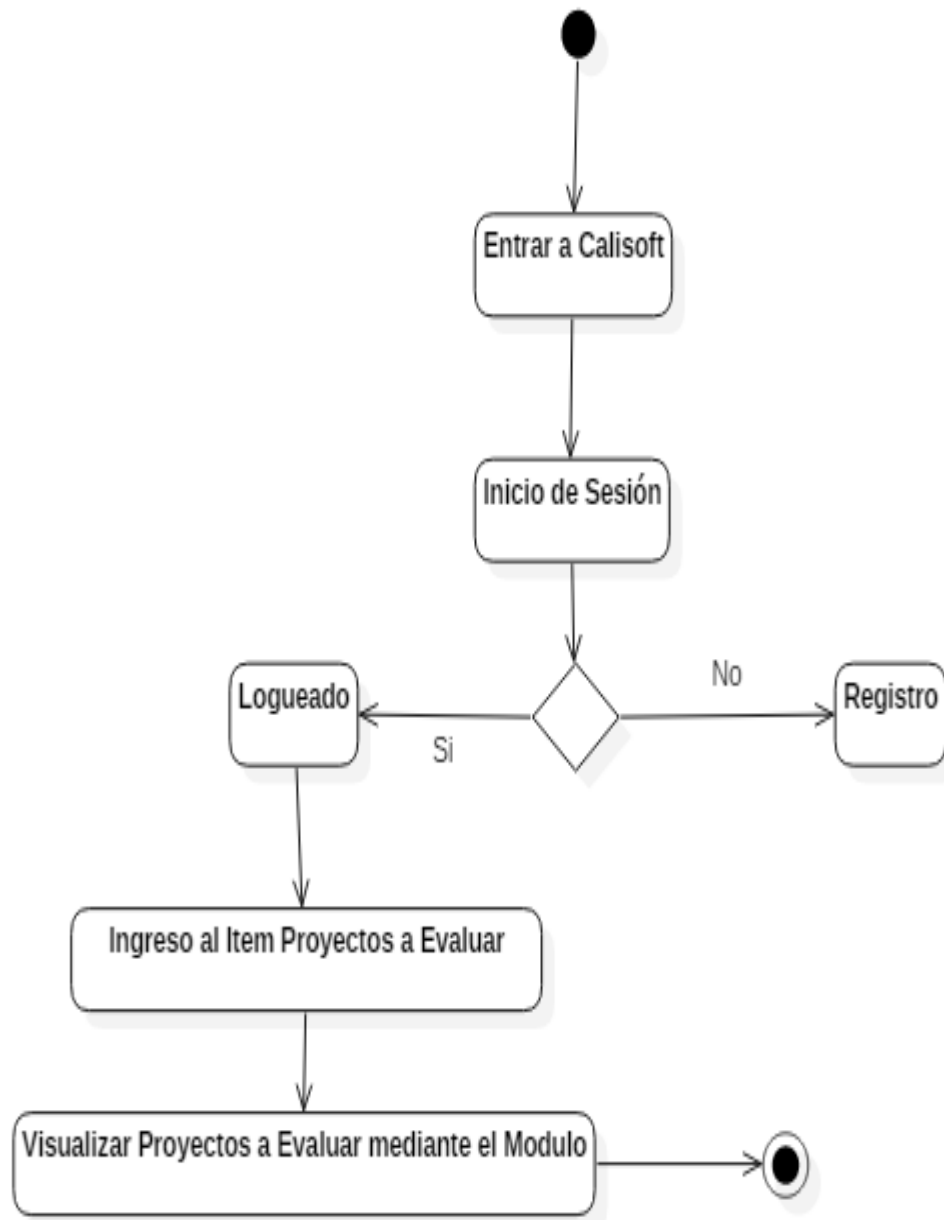
Imagen 20 Diagrama de Actividad Seleccionar Proyecto a Evaluar.
