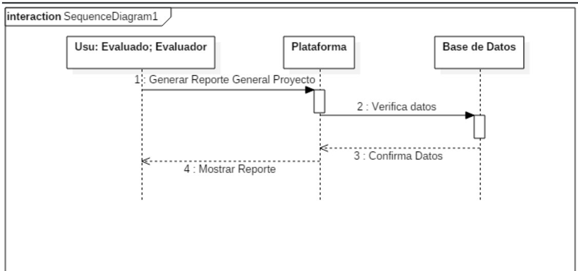
Imagen 14 Diagrama de Secuencia Reporte General de Estudiante, Evaluador Según Proyecto.
