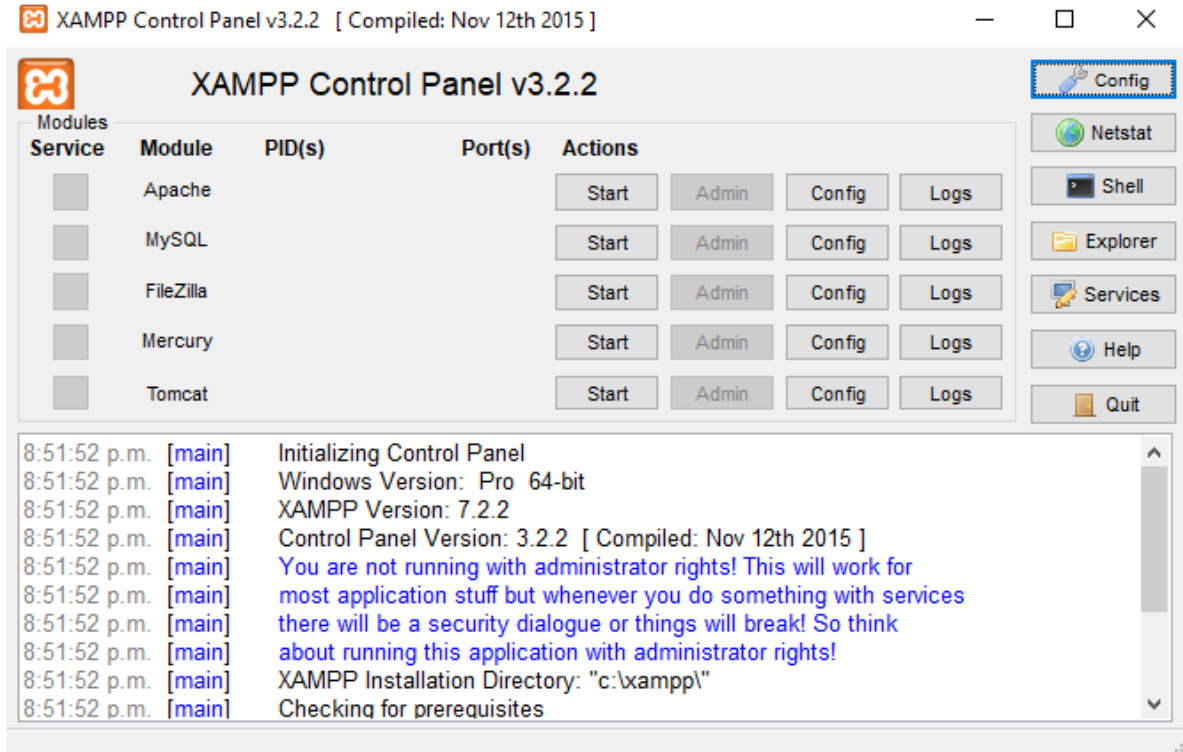
Ilustración 11 Interfaz XAMPP
