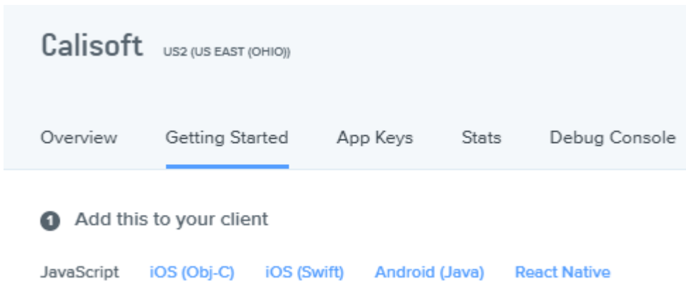
Ilustración 38 Pestañas Pusher
