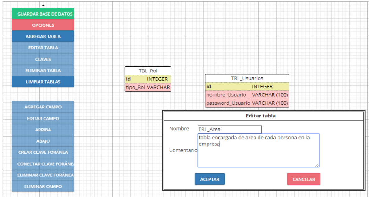
Imagen 47 Manejo de Tablas.
