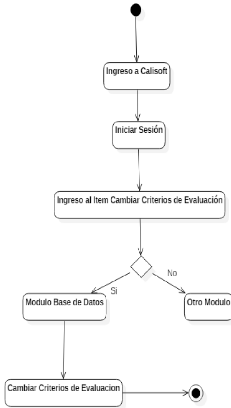
Imagen 24 Diagrama de Actividad Cambiar Criterios de Evaluación.
