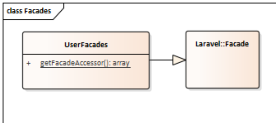
Figura 37 Diagrama de clases de usuarios facades.
