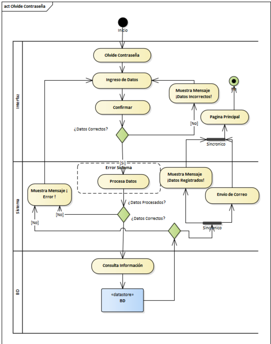
Figura 25 Diagrama de actividades de recuperar contraseña.
