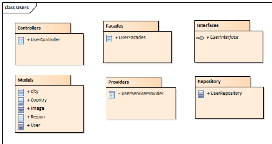
Figura 35 Menú Del diagrama de clases de usuarios.
