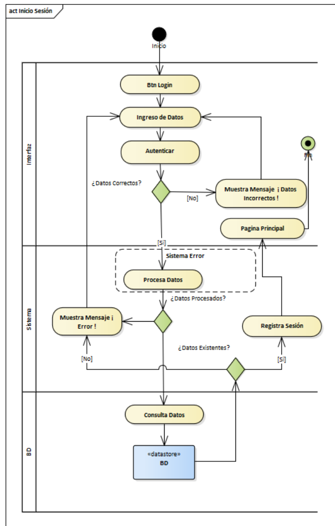
Figura 22 Diagrama de actividades de inicio de sesión.
