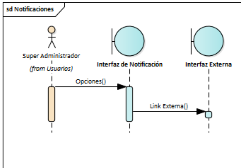
Figura 11 Diagrama de secuencia de notificaciones.
