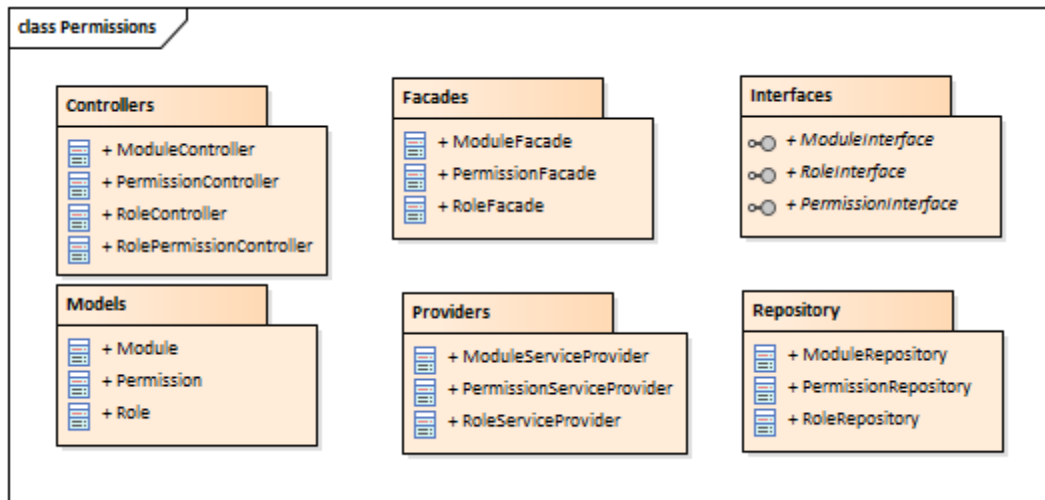
Figura 42 Diagrama de clases de menú de permisos.
