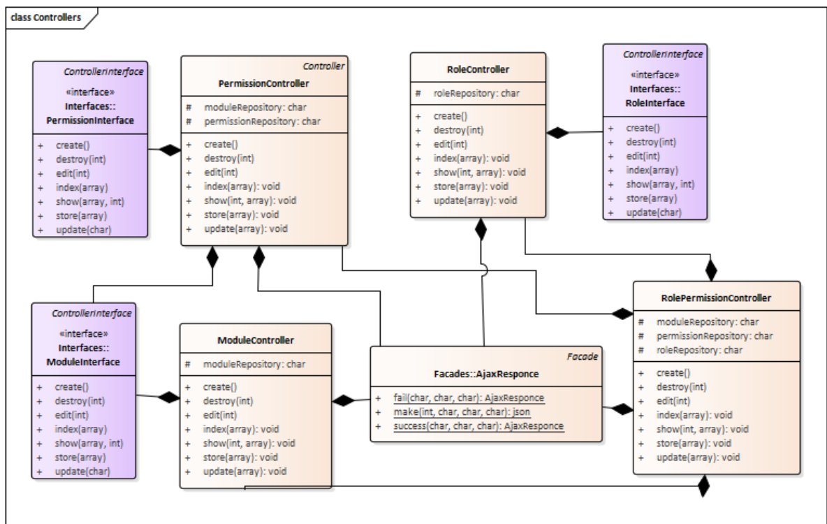
Figura 43 Diagrama de clases de permisos controllers.
