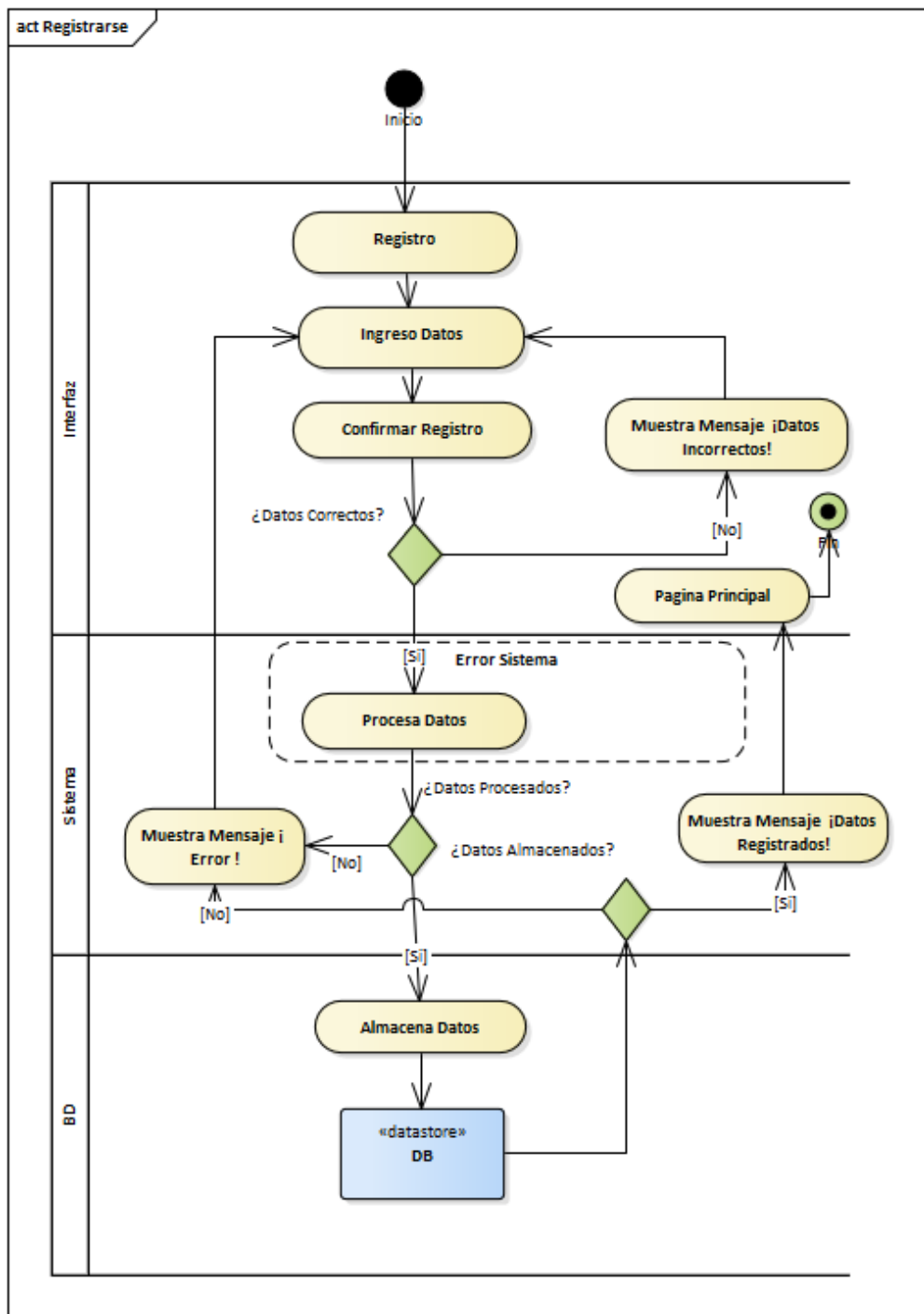
Figura 26 Diagrama de actividades de registrar datos.
