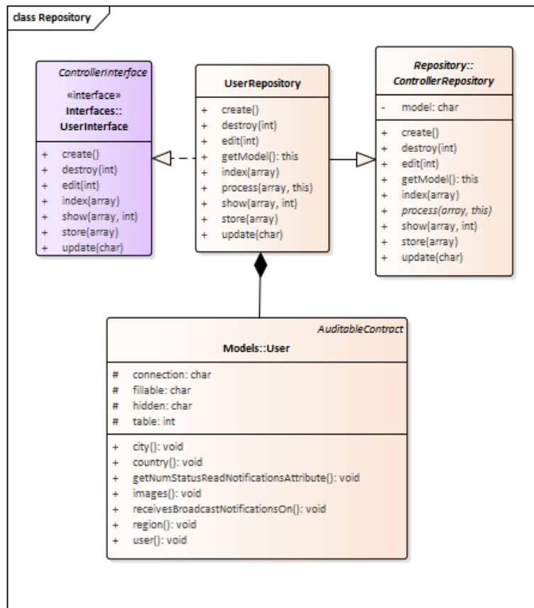
Figura 41 Diagrama de clases de usuarios repository.
