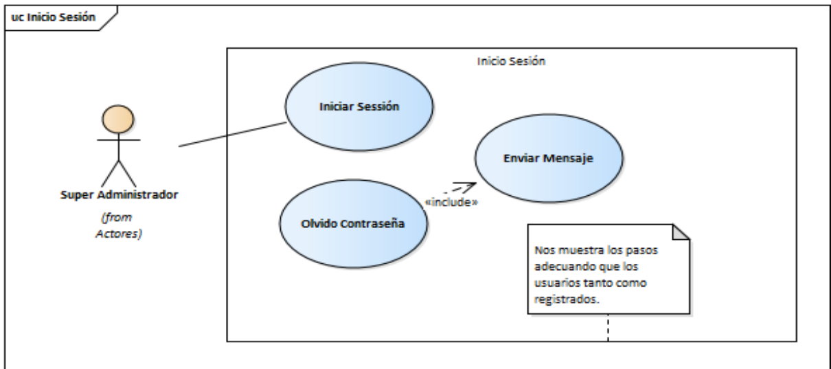
Figura 8 Diagrama de casos de uso de inicio de sesión.
