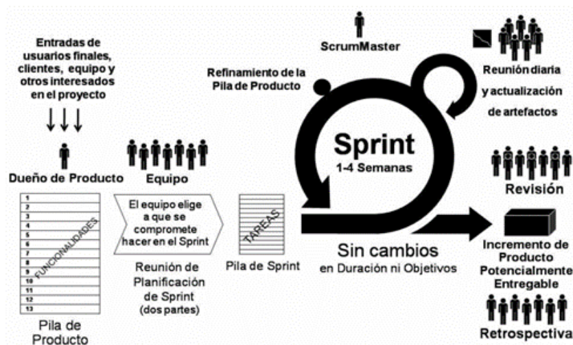
Figura. 3 Estructura del marco de trabajo ágil “SCRUM”
