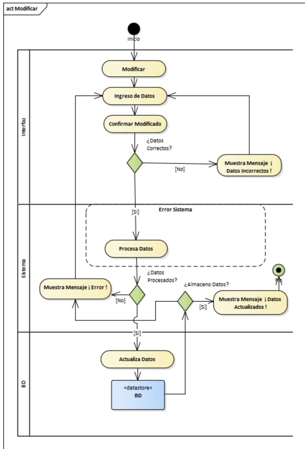
Figura 24 Diagrama de actividades de modificar perfil.
