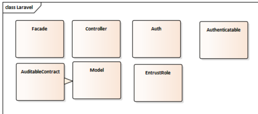
Figura 34 Diagrama de clases de laravel.
