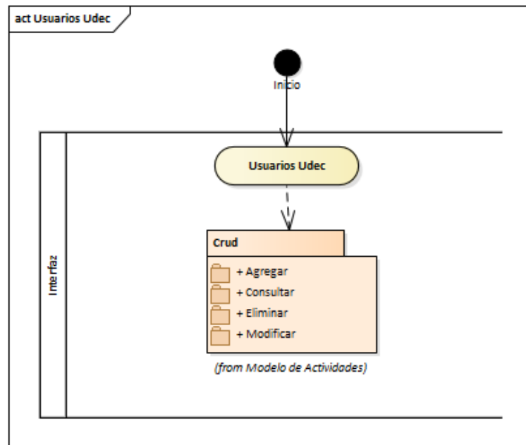
Figura 32 Diagrama de actividades de usuarios udec.
