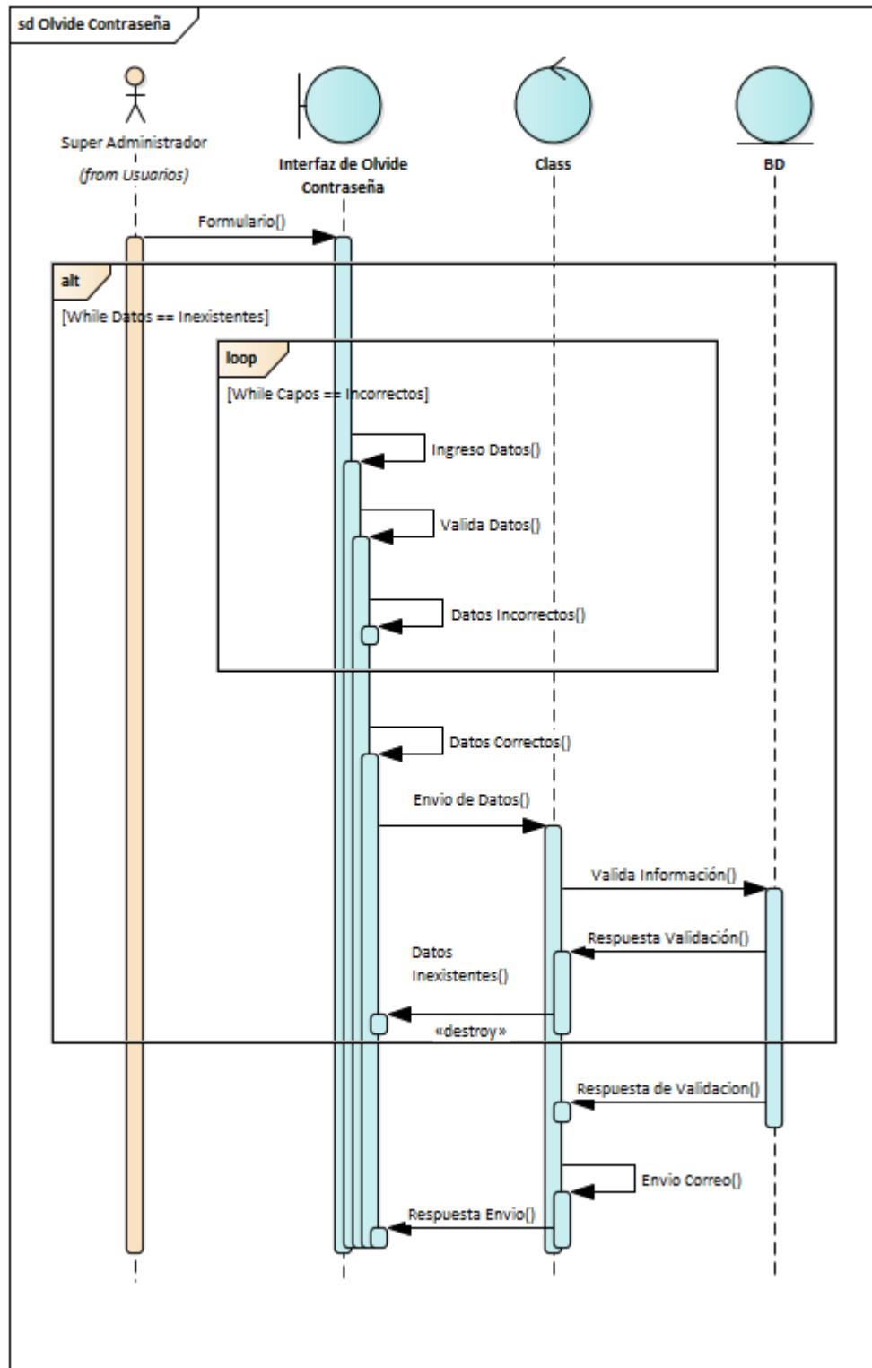
Figura 13 Diagrama de secuencia de recuperar contraseña.
