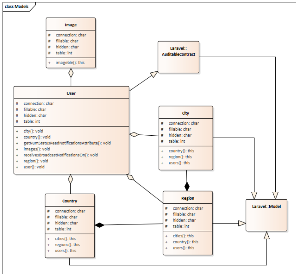
Figura 39 Diagrama de clases de usuarios models.
