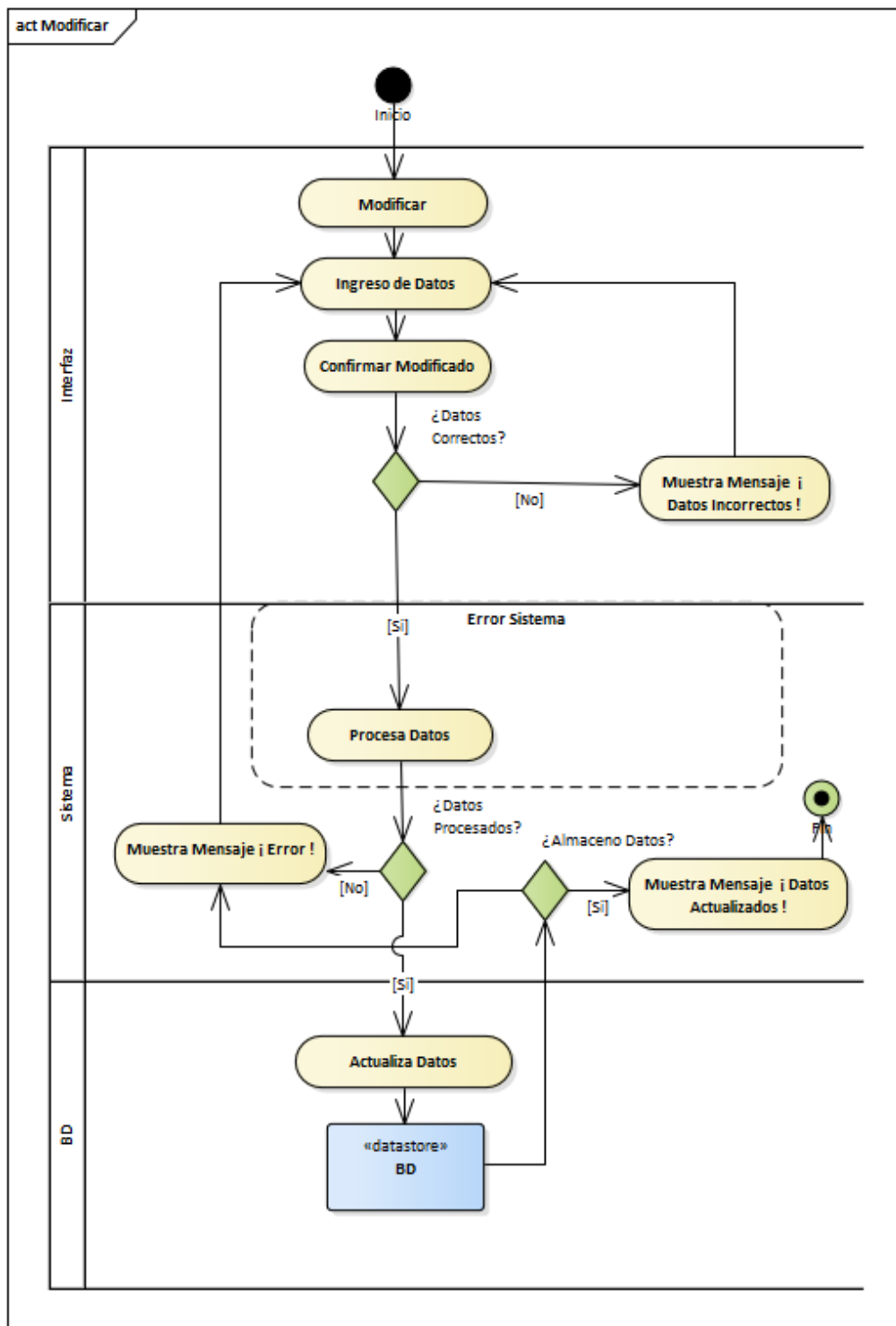
Figura 28 Diagrama de actividades de modificar datos.
