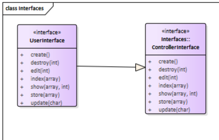
Figura 38 Diagrama de clases de usuarios interfaces.
