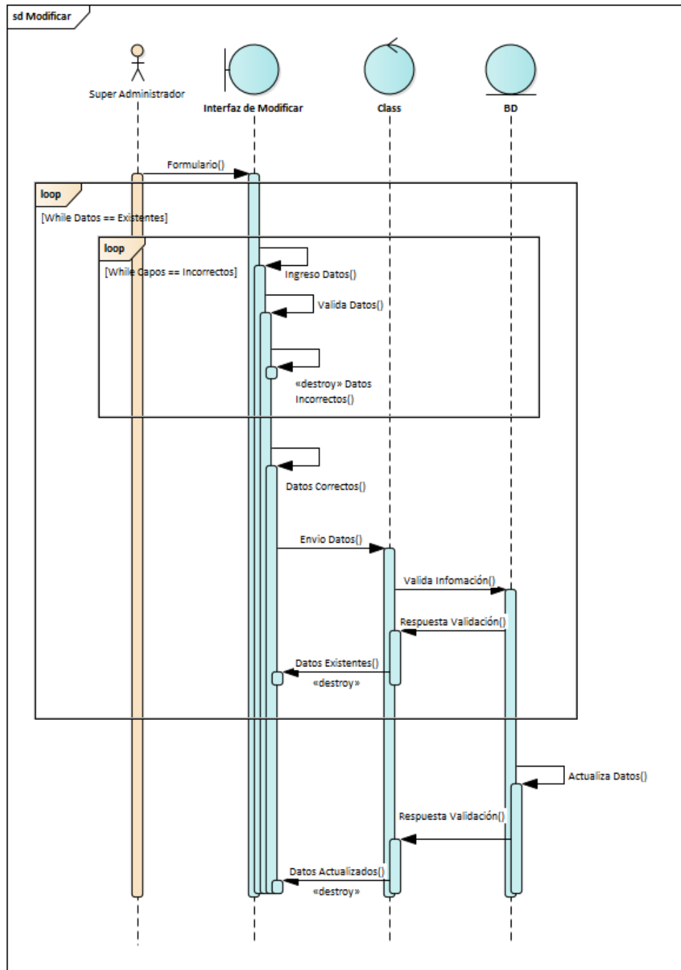
Figura 12 Diagrama de secuencia de modificar perfil.
