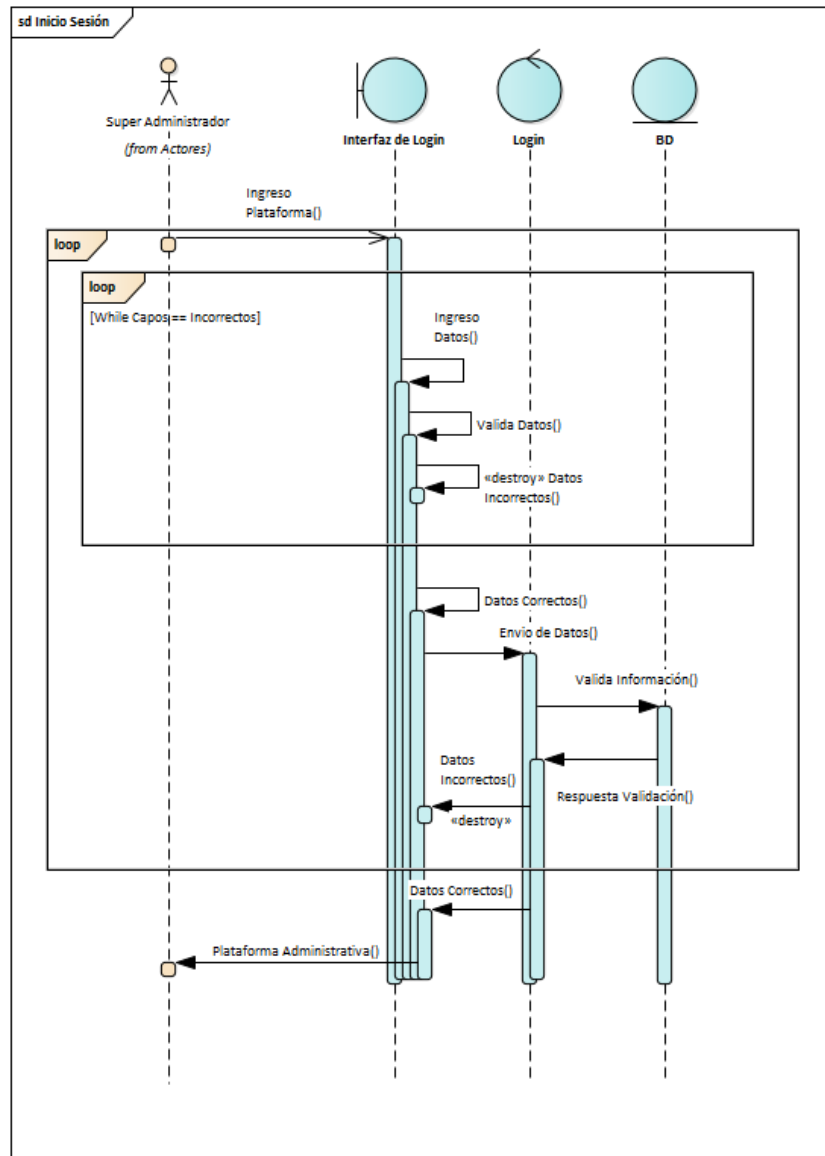
Figura 9 Diagrama de secuencia de inicio de sesión.
