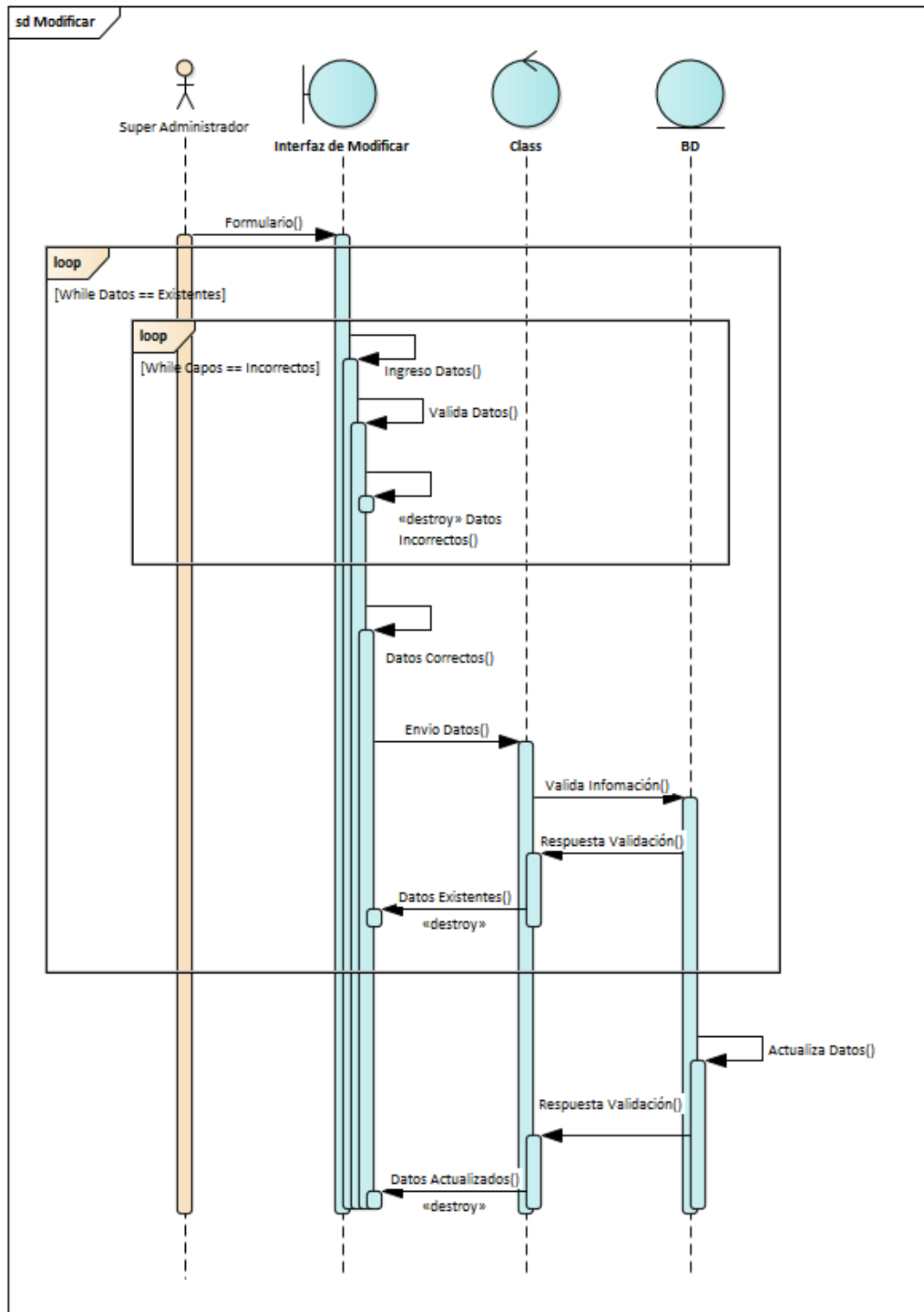
Figura 16 Diagrama de secuencia de modificar datos.
