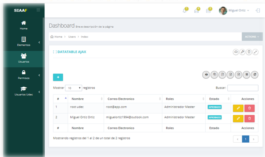
Figura 128 Enlace para la edición de usuario
