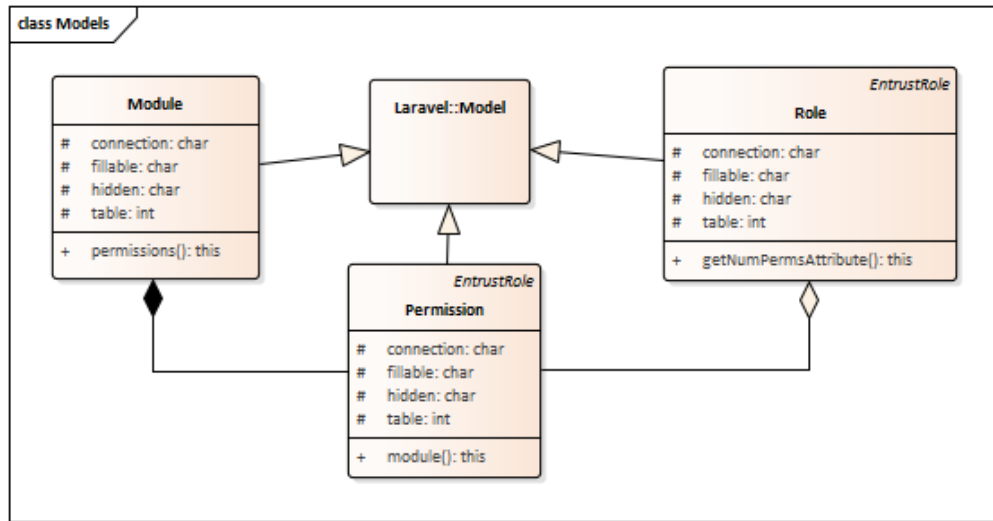
Figura 46 Diagrama de clases de permisos models.
