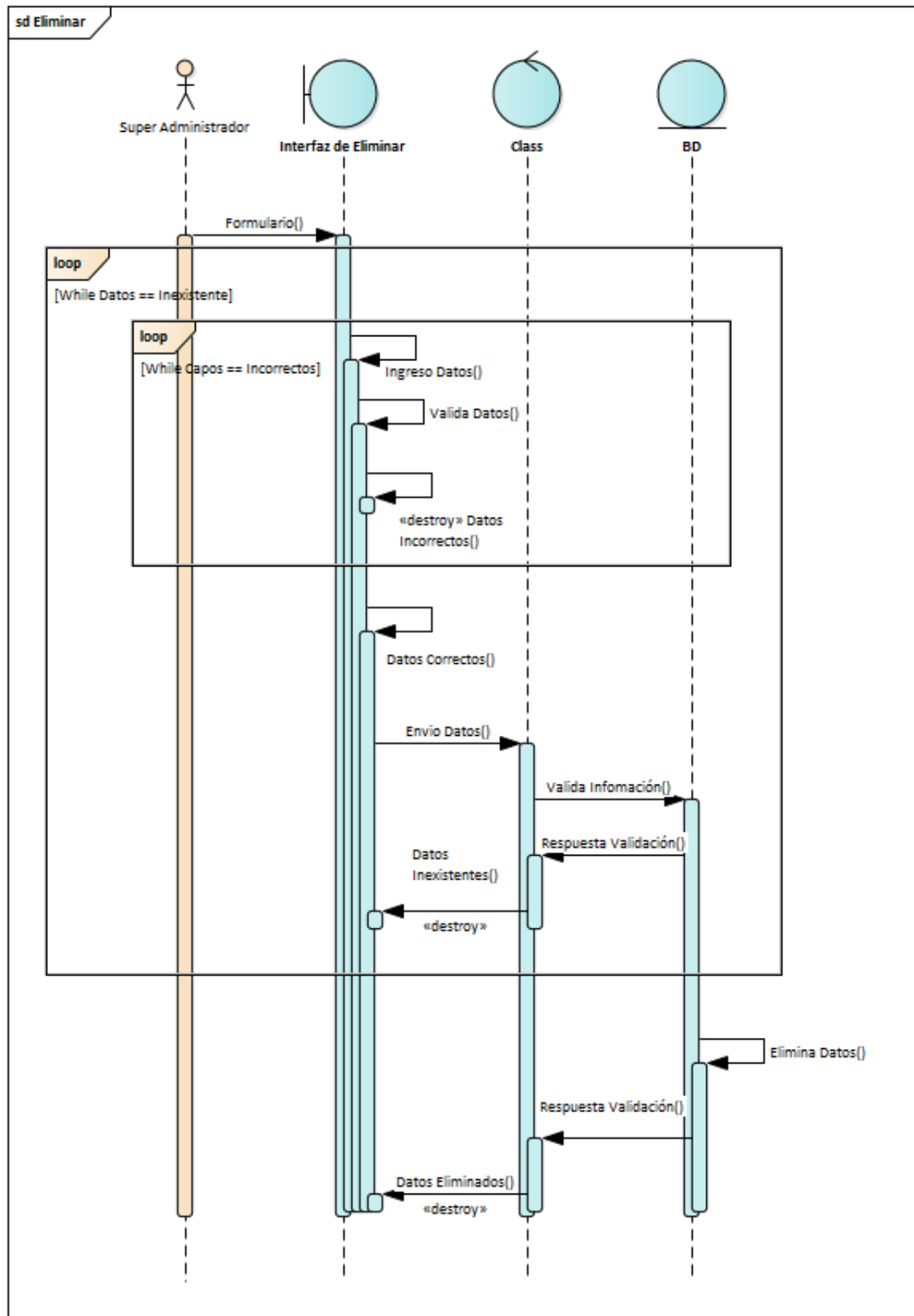
Figura 18 Diagrama de secuencia de eliminar datos.
