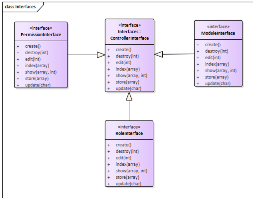
Figura 45 Diagrama de clases de permisos interfaces.
