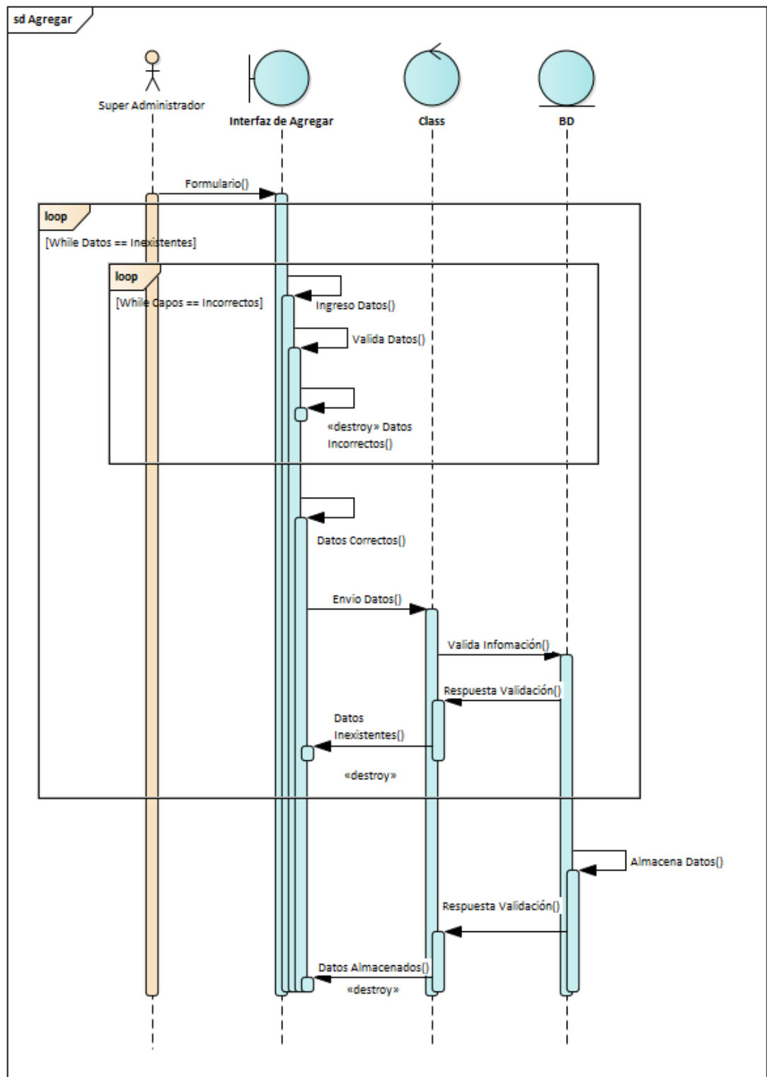
Figura 15 Diagrama de secuencia de agregar datos.
