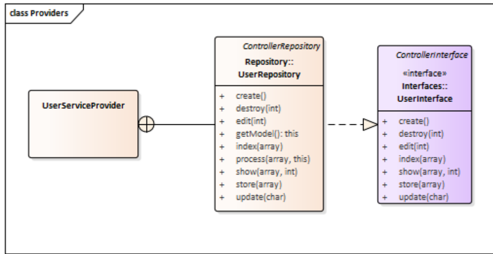
Figura 40 Diagrama de clases de usuarios providers.
