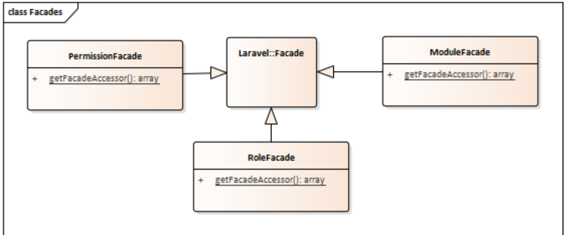
Figura 44 Diagrama de clases de permisos facades.
