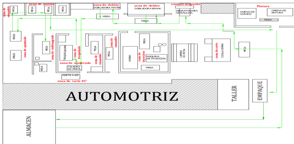
PLANO 4: DIAGRAMA DE RECORRIDO PLANTA DE DIVISIÓN CONSTRUCCIÓN
