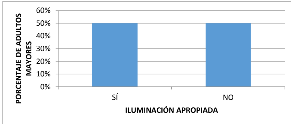
Gráfica 29. Distribución porcentual de la iluminación.
