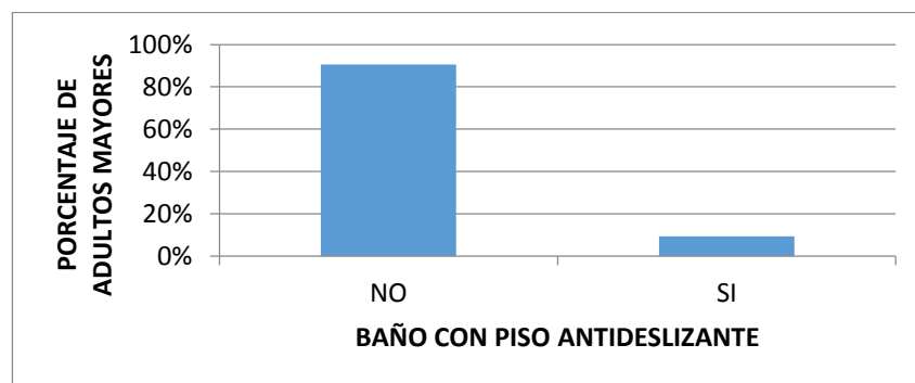
Gráfica 25. Distribución porcentual de la presencia de piso antideslizante en los baños.
