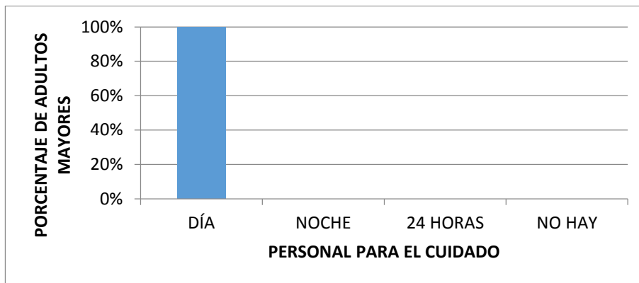
Gráfica 31. Distribución porcentual de la presencia de personal para el cuidado
