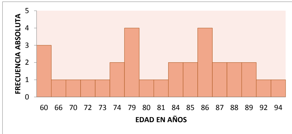
Gráfica 2. Histograma de frecuencias para la distribución de la edad
