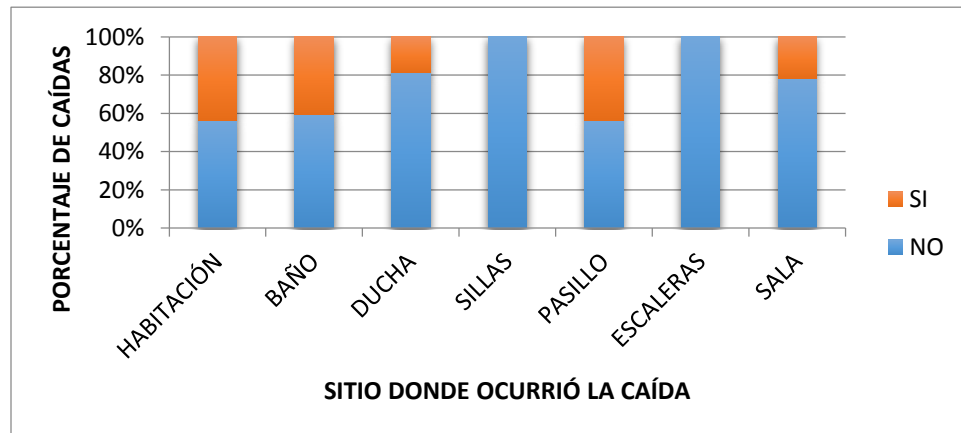
Gráfica 9. Porcentaje de los sitios en donde el adulto mayor presento la caída.
