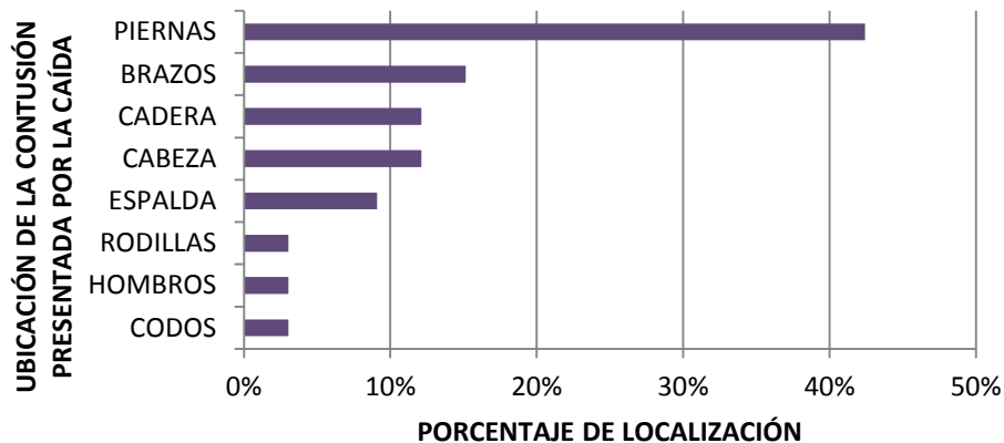
Gráfica 33. Porcentaje de localización corporal de las contusiones presentadas como consecuencia de las caídas.
