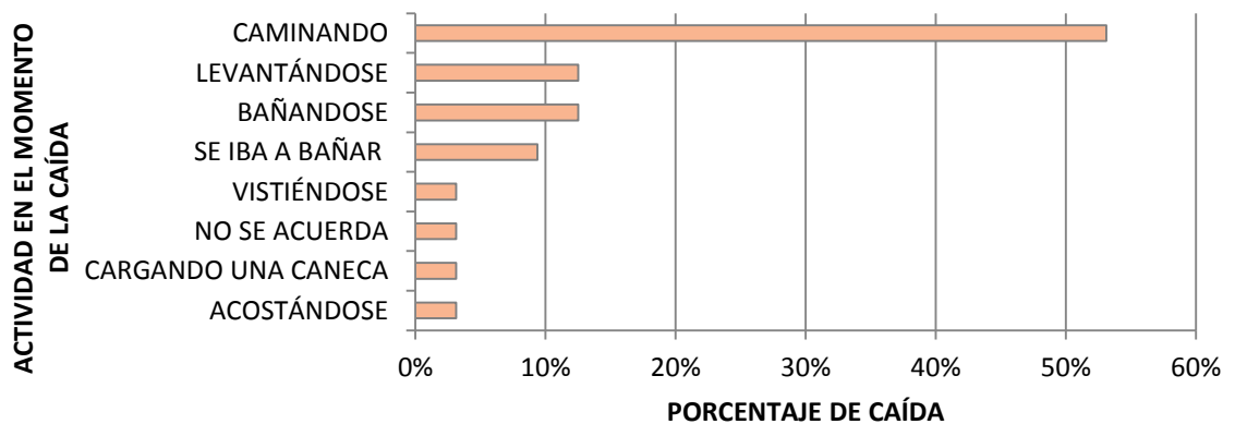
Gráfica 22. Porcentaje de caídas durante la realización de diferentes actividades.
