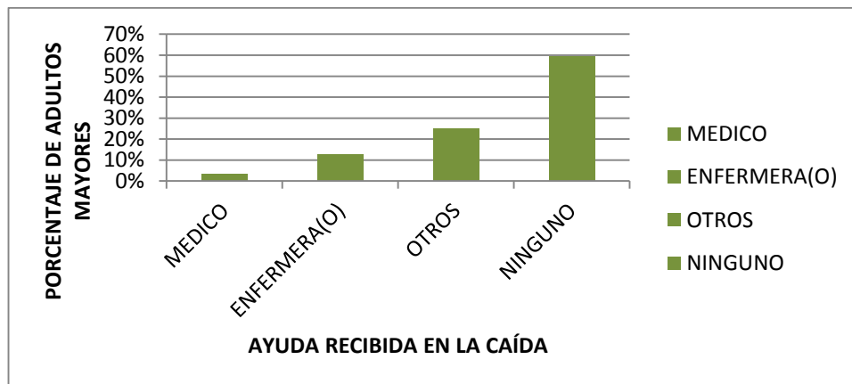
Gráfica 10. Distribución porcentual de la ayuda recibida luego de presentar la caída.
