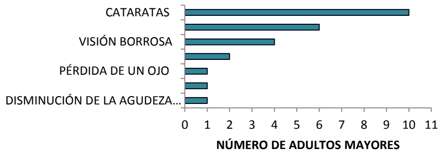
Gráfica 14. Frecuencia absoluta de alteraciones oculares.
