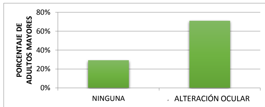
Gráfica 13. Distribución porcentual de alteración ocular.
