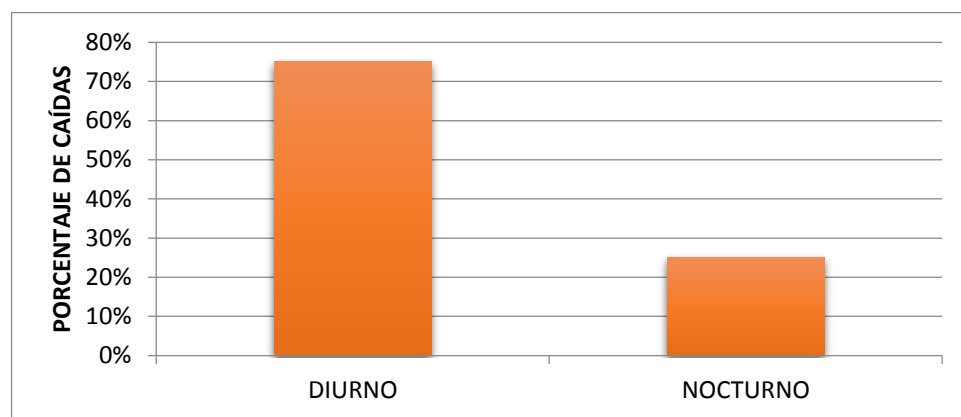
Gráfica 7. Distribución porcentual de la presencia de caídas según la jornada.
