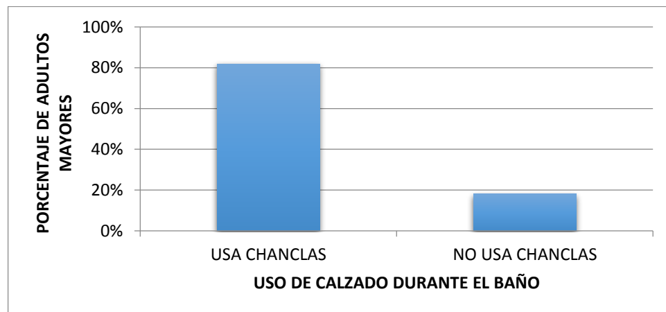
Gráfica 17. Distribución porcentual del uso de chanclas durante el baño.
