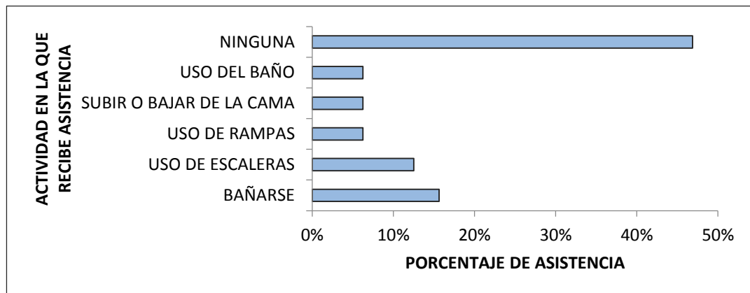
Gráfica 23. Distribución porcentual de los adultos mayores que reciben asistencia o ayuda en la realización de diferentes actividades que implican riesgo de caída.
