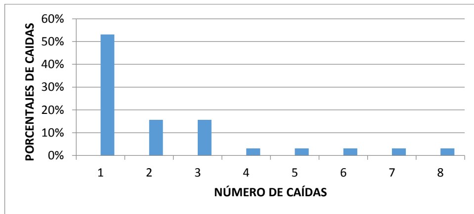
Gráfica 4. Porcentaje del número de caídas presentadas
