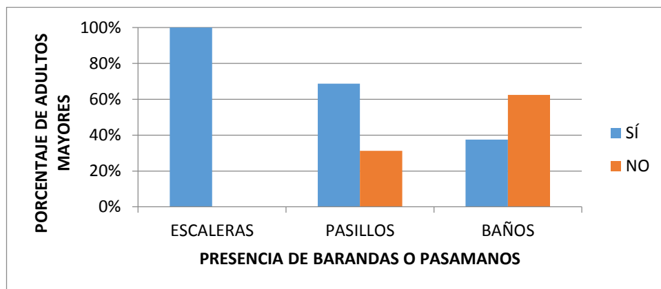
Gráfica 30. Distribución porcentual de la presencia de barandas o pasamanos.
