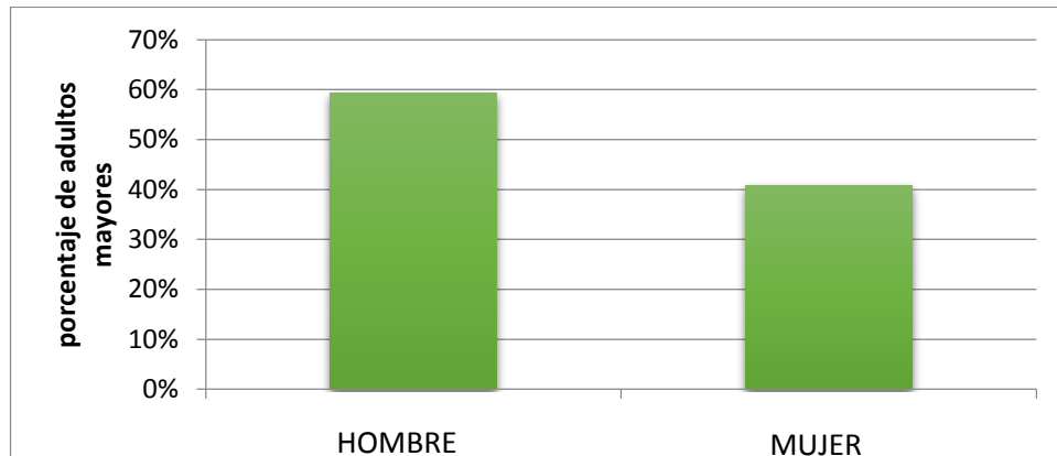
Gráfica 3. Distribución porcentual de las caídas por sexo
