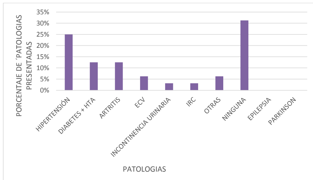
Gráfica 12. Distribución porcentual de las patologías presentadas.
