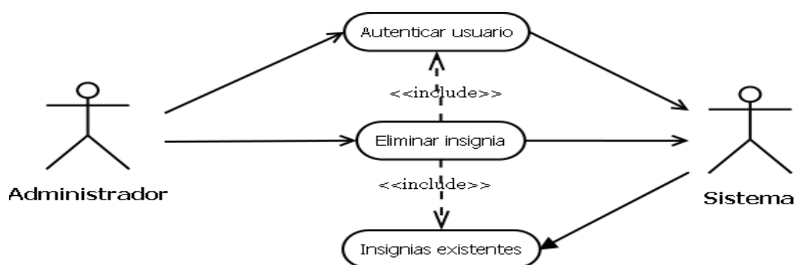
Ilustración 21 Caso de uso: Eliminar insignia
