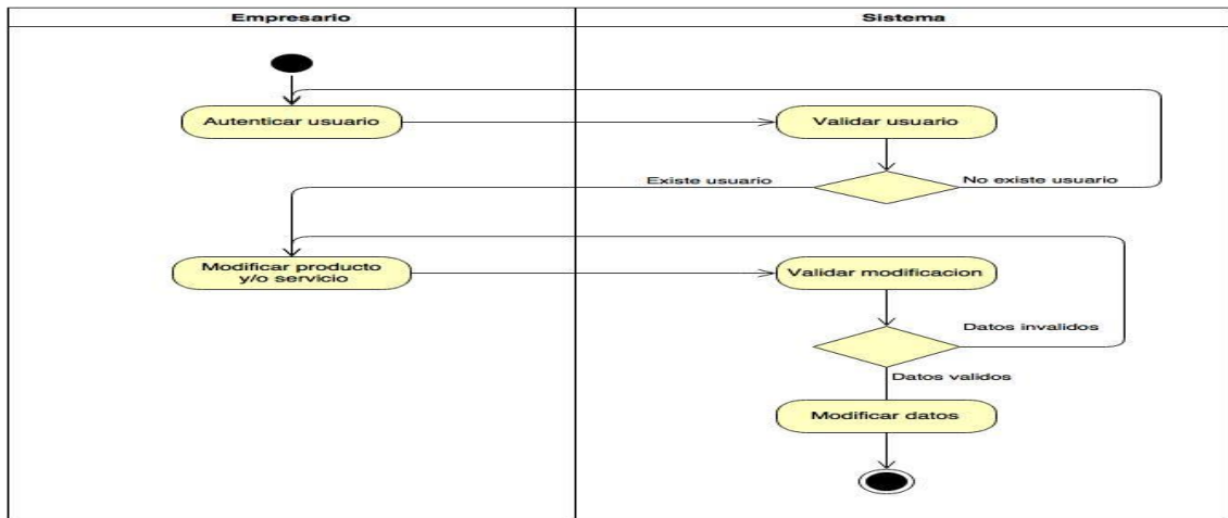
Ilustración 30 Diagrama de actividad: Modificar producto y/o servicio
