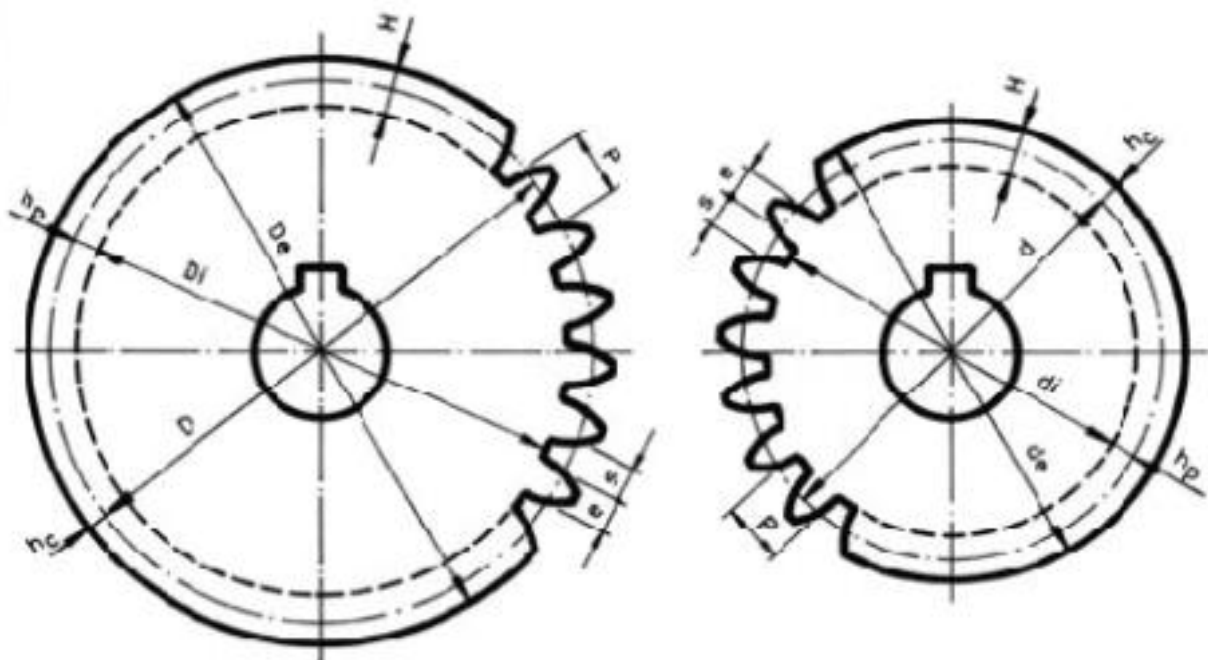
Figura. 5.6 Corona y Piñón [26].
