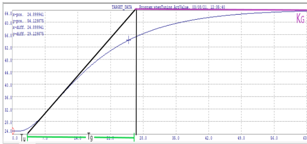
Figura. 6.14 Implementación del método “CHR”.
