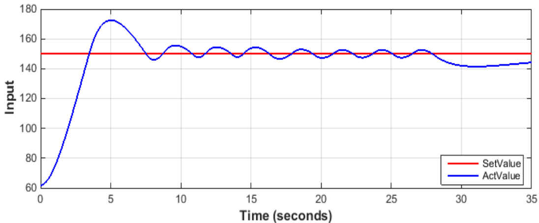
Figura. 6.17 Representación de la oscilación periódica.
