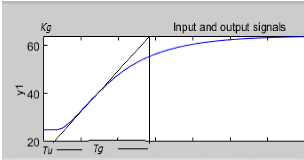
Figura. 6.13 Señal tipo “s” o sigmoideal
