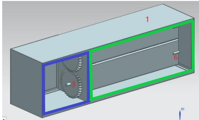
Figura. 5.4 Diseño de la Ventila en 3D, parte frontal.
