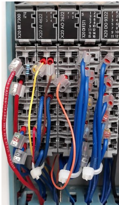
Figura. 6.6 Módulos.
