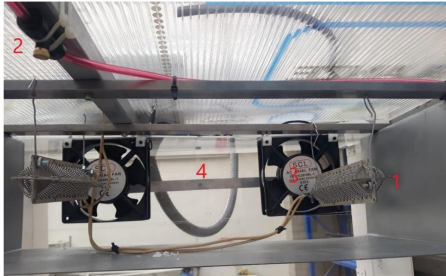
Figura 7.3 Actuadores de los sistemas.
