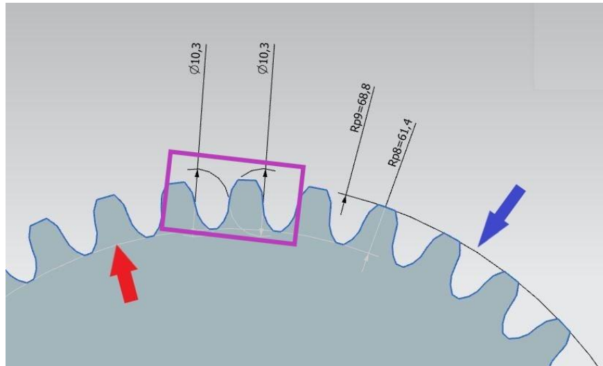
Figura. 5.7 Dientes del engrane.
