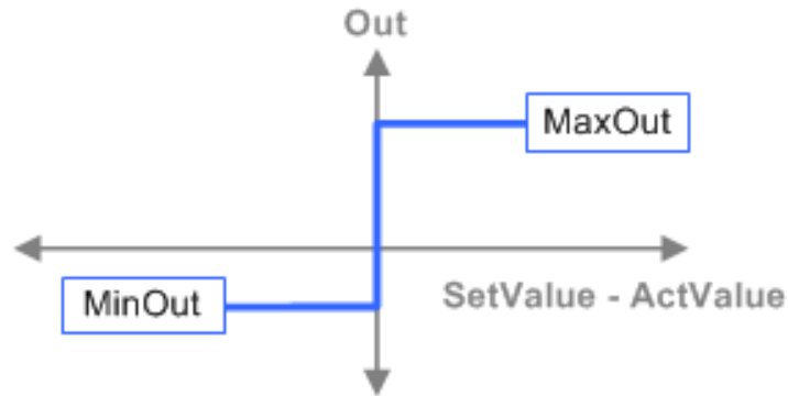
Figura. 6.16 Ajuste mínimo y máximo al actuador.
