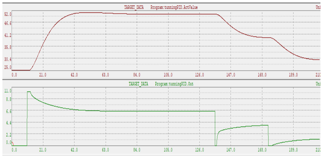
Figura. 7.4 Respuesta del PID.
