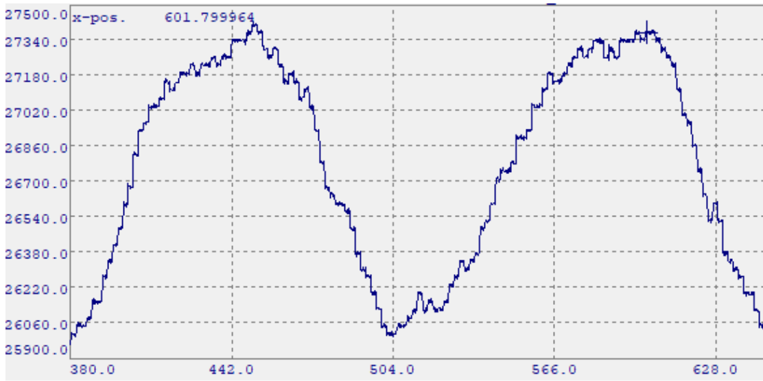
Figura 6.19 Valles o crestas de la oscilación periódica.
