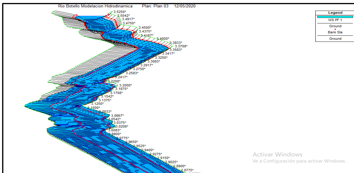
Gráfica 42: Perfil del tramo 3 del río Botello parte baja. Fenómeno de la niña año 2009 inundaciones ocasionadas por los grandes caudales.
