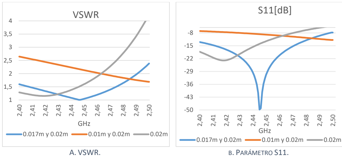
GRÁFICA 6. PARÁMETROS ANTENA YAGI-UDA TRAS VARIAR LA SEPARACIÓN LOS DIRECTORES
