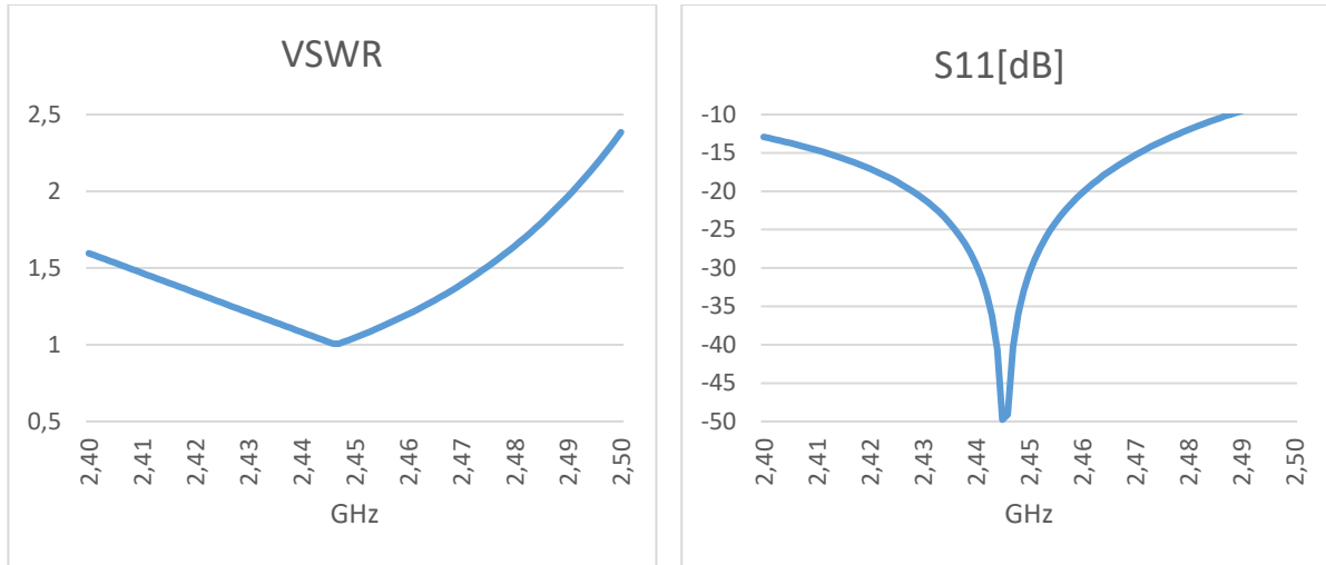
A. VSWR.
