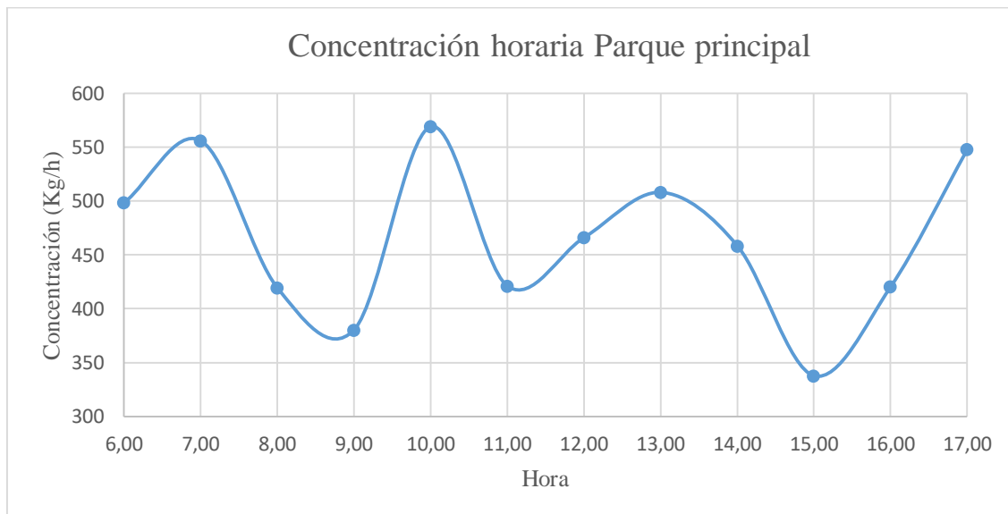
Figura 30. Concentración horaria de CO 2 para la vía Parque Principal. Fuente: Autores, 2019
