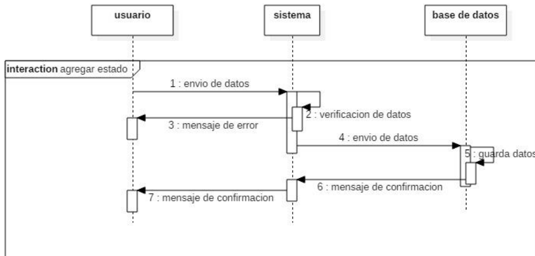
Figura 24 Diagrama de secuencia agregar estado
