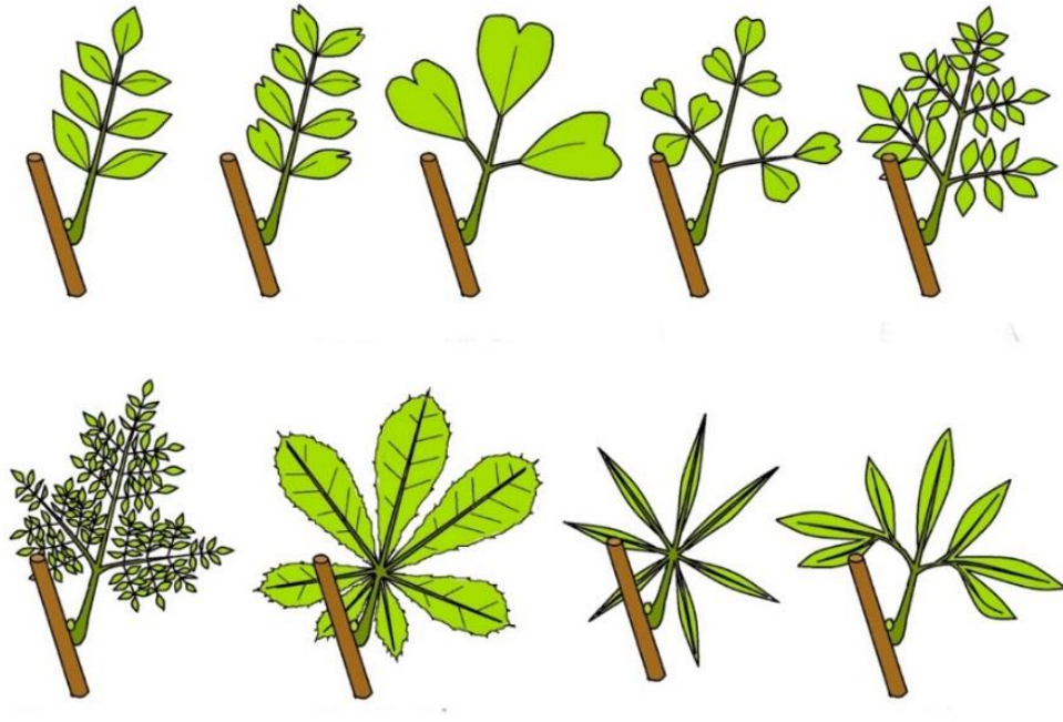
Figura 5. Hojas compuestas
