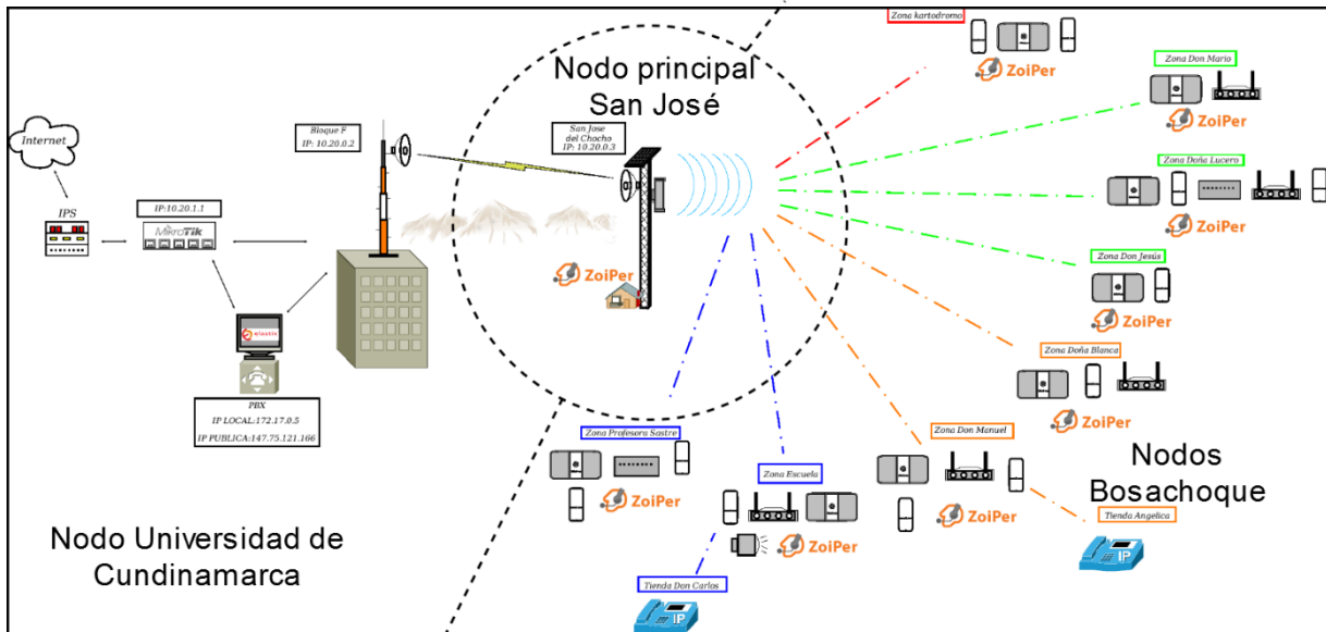
Figura 1. Infraestructura física de la red comunitaria en Bosachoque 2018.
