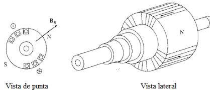
Figura . Rotor de polos no salientes en una máquina sincrónica
