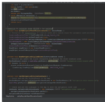
ILUSTRACIÓN 24: TARJETAS INDIVIDUALES.
