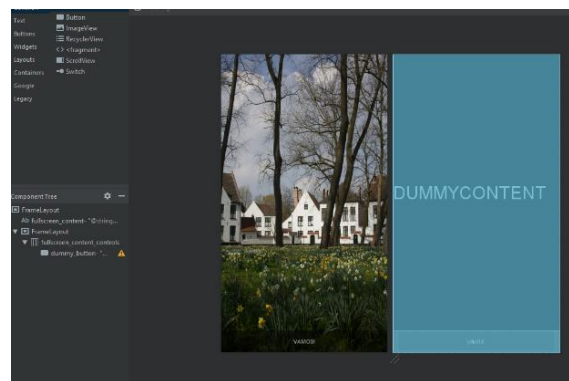
ILUSTRACIÓN 17: INTERFAZ
