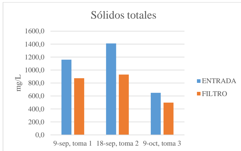
Gráfica 9. Relación de sólidos totales en entrada y filtro, Autoras.
