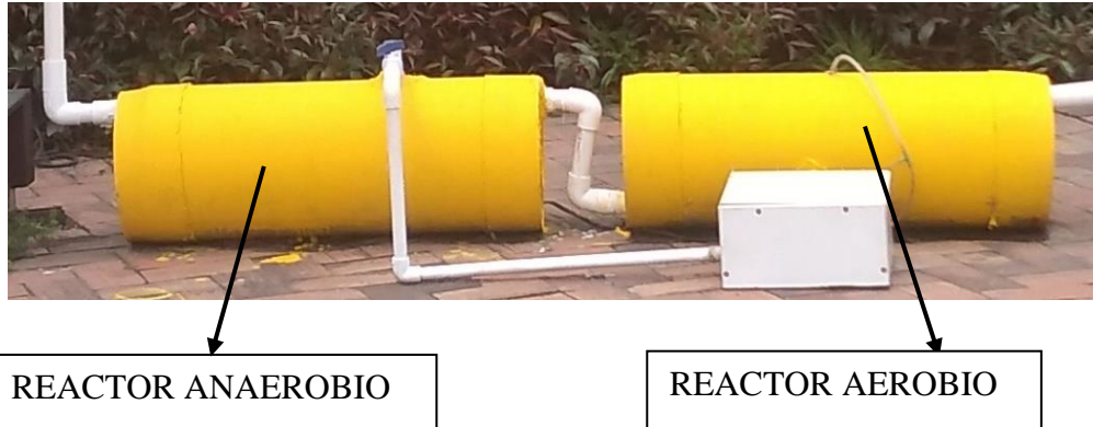
Imagen a. Reactores anaerobio y aerobio, Autoras.
