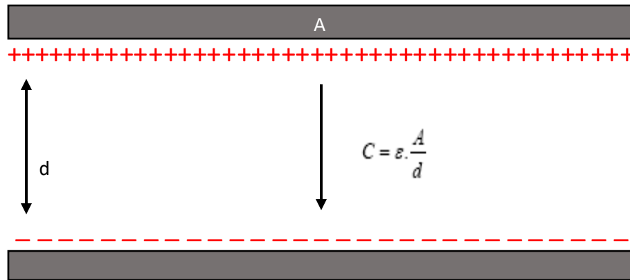
Fig. 10. Placas paralelas
