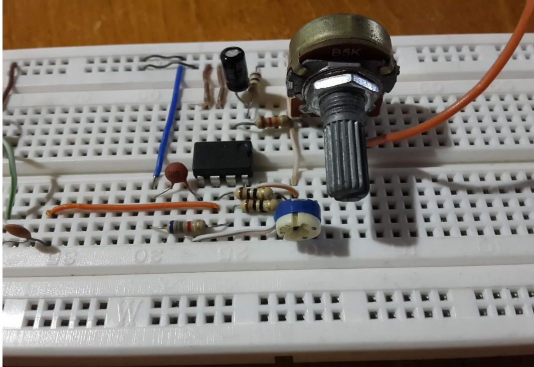
Fig. 9. Montaje circuito LM331 físico
