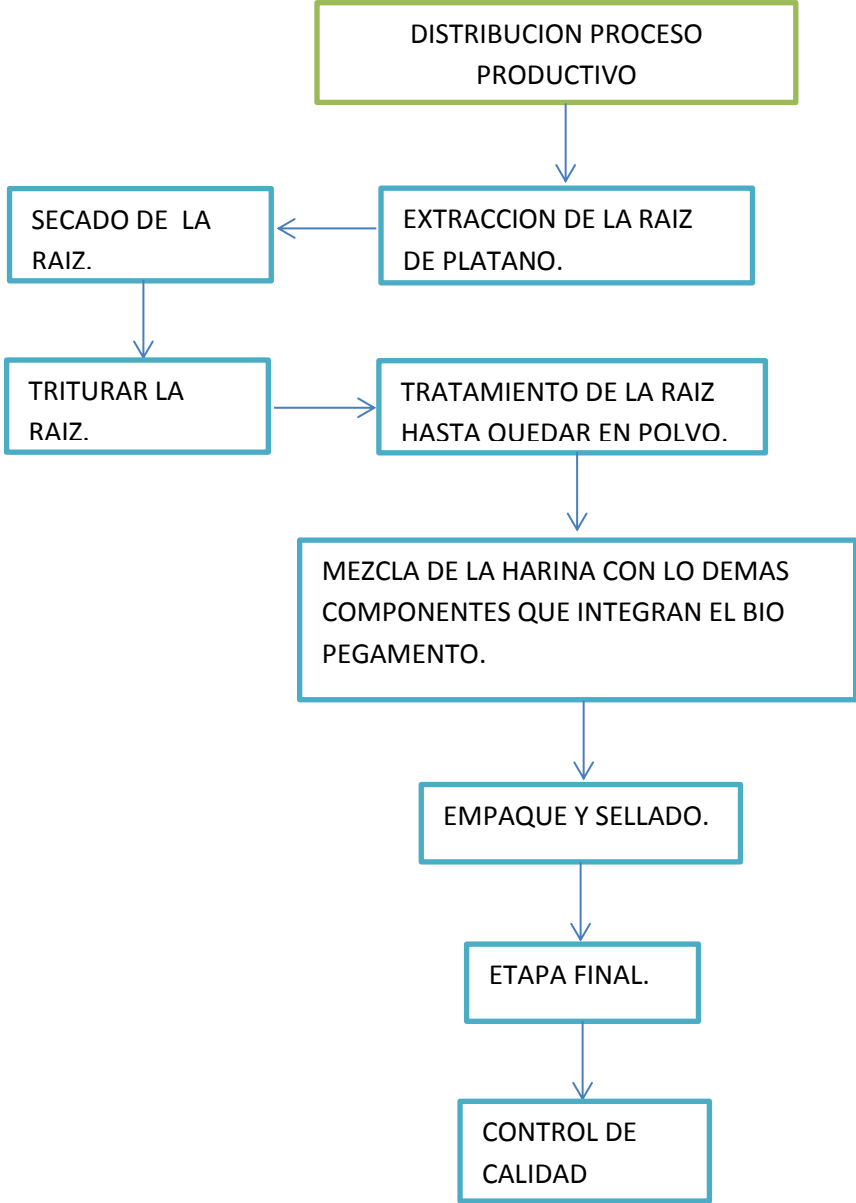
Figura 8. Distribución proceso productivo
