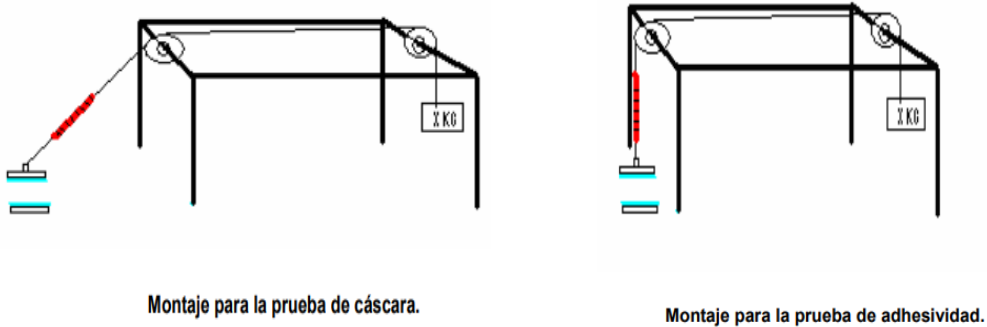
Figura 2. Montaje para pruebas de calidad
